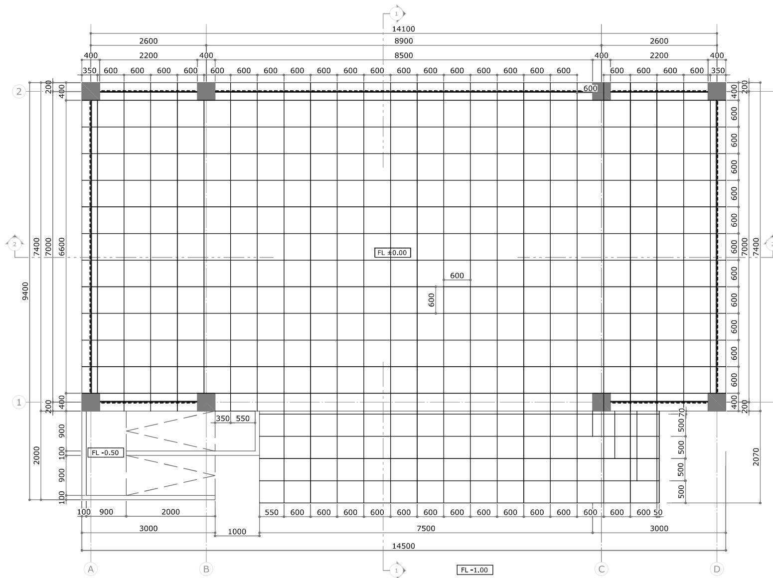
DENAH POLA LANTAI 1:30
