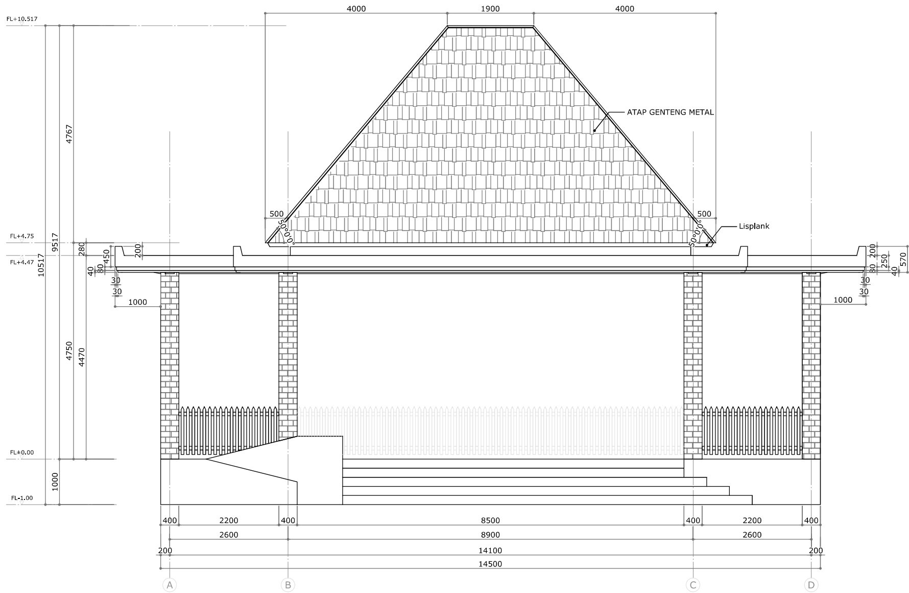
T. DEPAN 1:30
