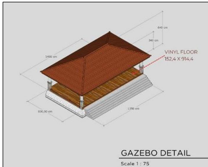
Gambar 18. Desain bangunan fungsi panggung
