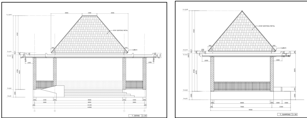
Gambar 4. Gambar Renc. Panggung Balai Warga
