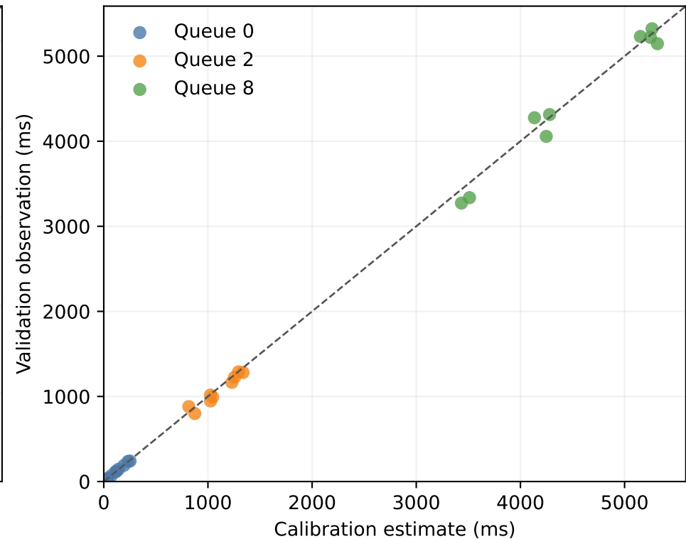
p95 TTFT
