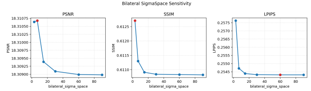
图 7. 双边滤波空间域参数变化对平均指标的影响。
