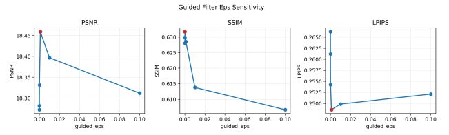
图 10. 引导滤波正则参数变化对平均指标的影响。
