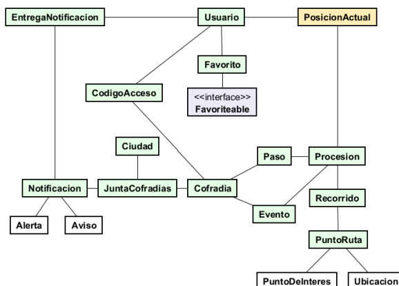
Figura 4.3: Diagrama de dominio simplificado, referido a las colecciones de Firestore
