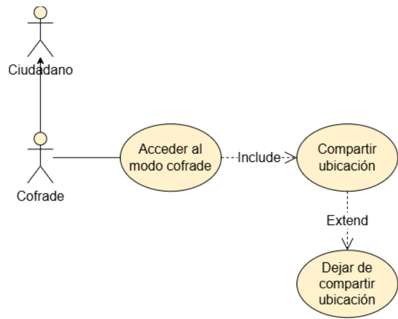
Figura 3.2: Diagrama de caso de uso Cofrade
