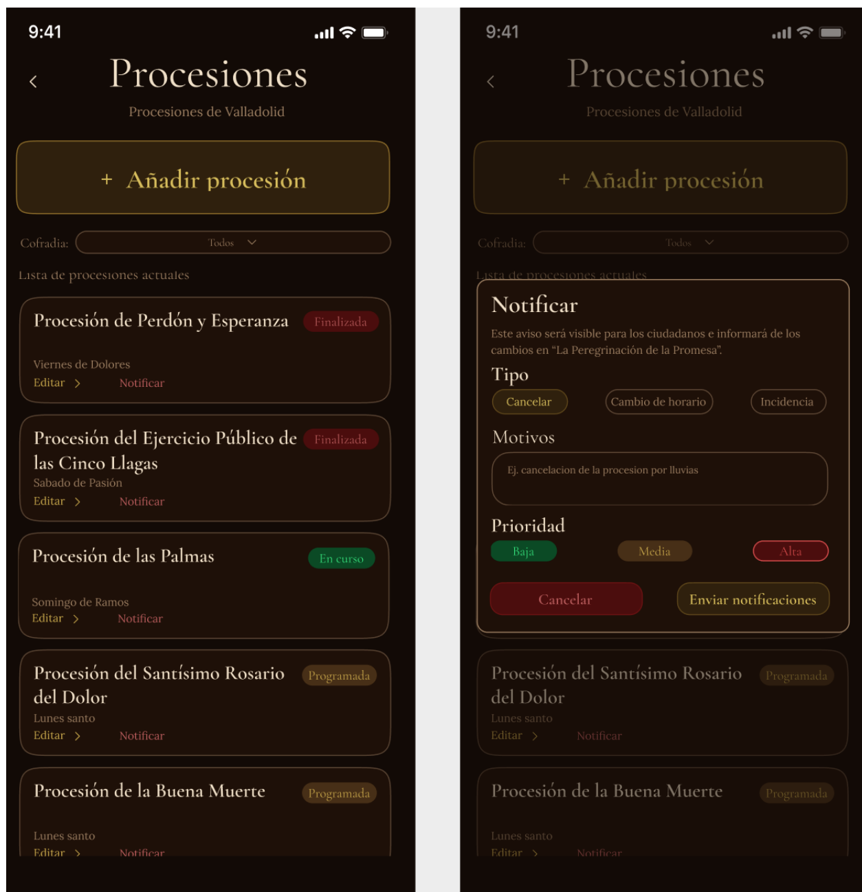
Figura 4.22: Mockup del listado de procesiones y del envío de una notificación
