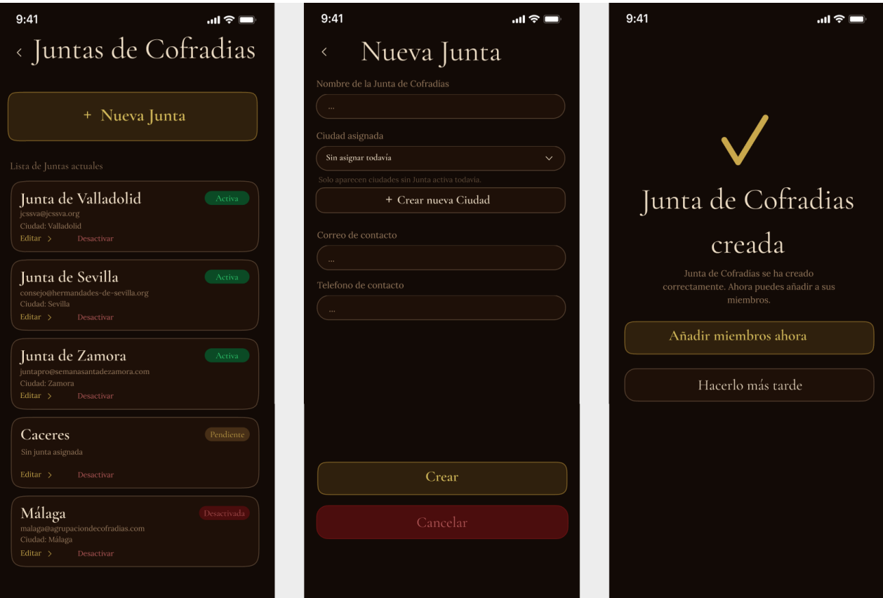
Figura 4.30: Mockup del listado de Juntas de Cofradías y de su creación
