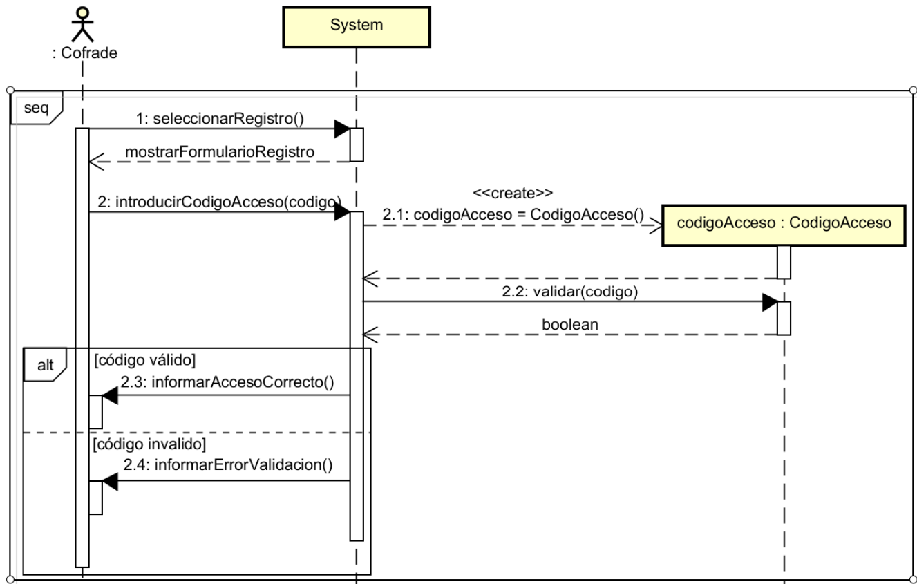
Figura 3.8: Diagrama de secuencia del CU “Acceder al modo cofrade”
