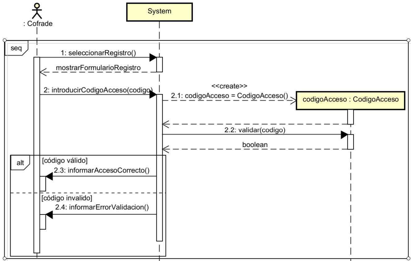
Figura 4.8: Diagrama de secuencia del CU “Acceder al modo cofrade”
