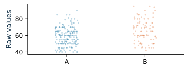
a Heart failure · age
