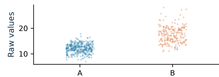
c WDBC · mean radius
