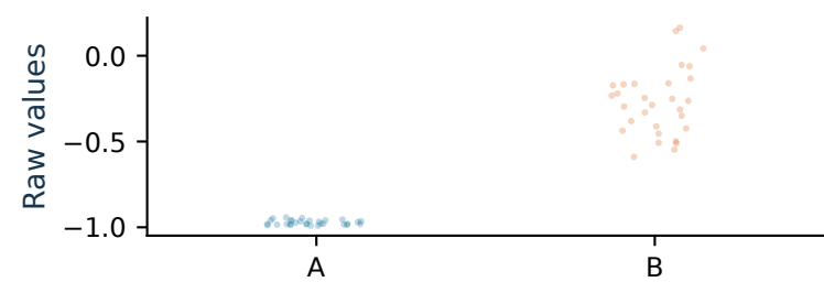
b Smartphone HAR · acceleration SD
