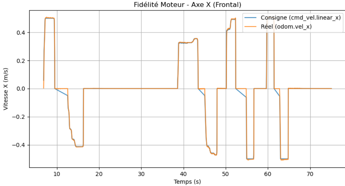
FIGURE 3 – Suivi de vitesse sur l'axe X (frontal) . L'écart au démarrage correspond aux 17,3 ms de temps de réaction initial. Les variations en cours de mouvement traduisent le glissement naturel des galets.
