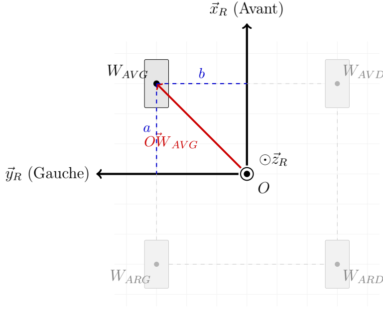
FIGURE 8 – Paramétrage géométrique du repère local du robot.
