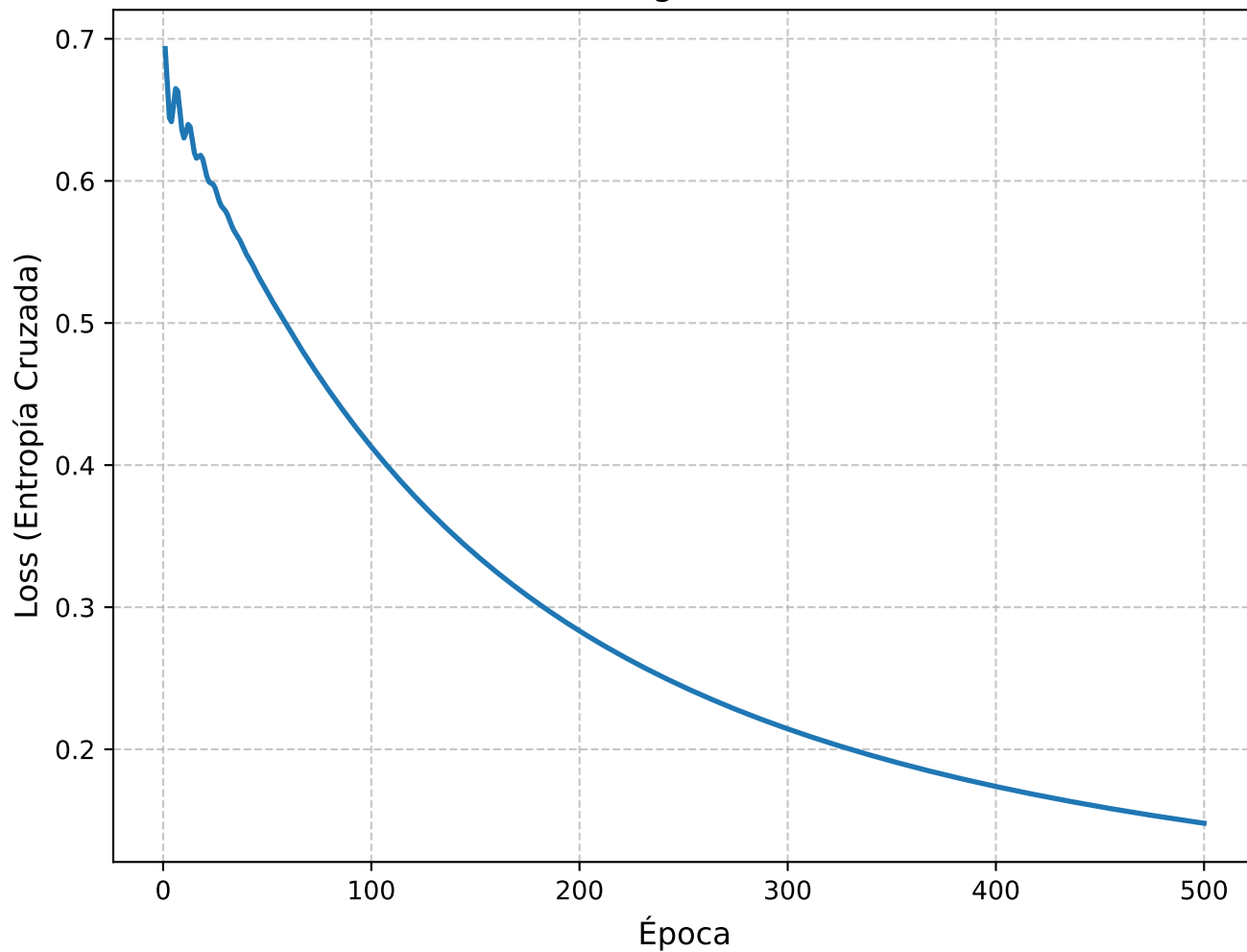
Curva de Convergencia (mGD) - MDE
