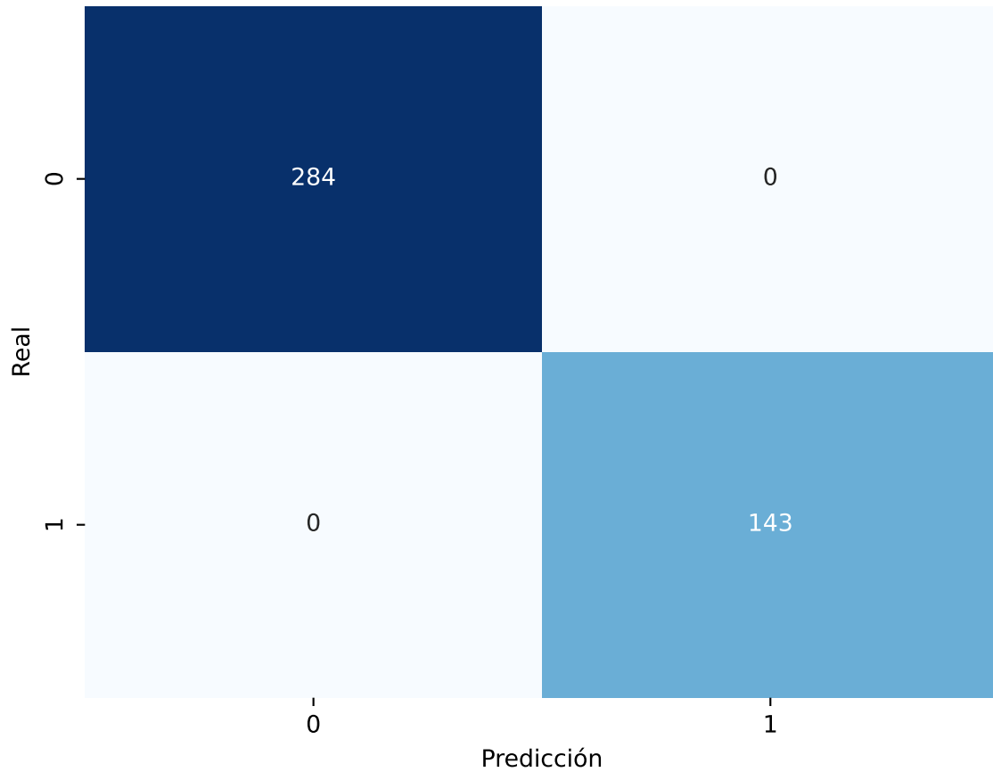
Matriz de Confusión - Train
