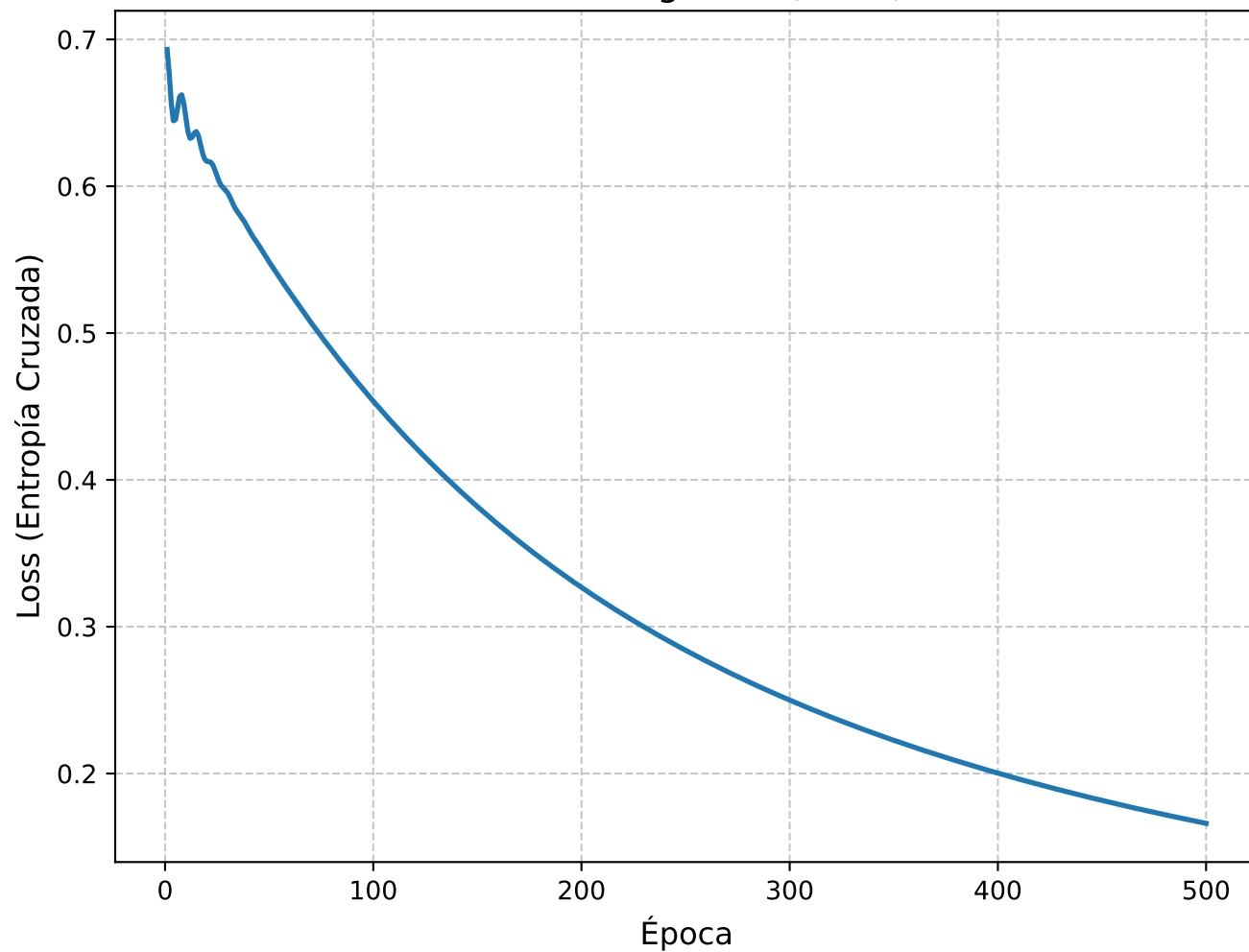
Curva de Convergencia (mGD) - MPE
