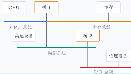
四总线结构
