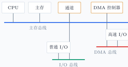
三总线结构
