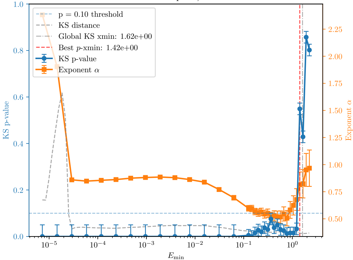
L-BFGS 200x200 10 samples \gamma : 0.14 - 0.55 L=200
