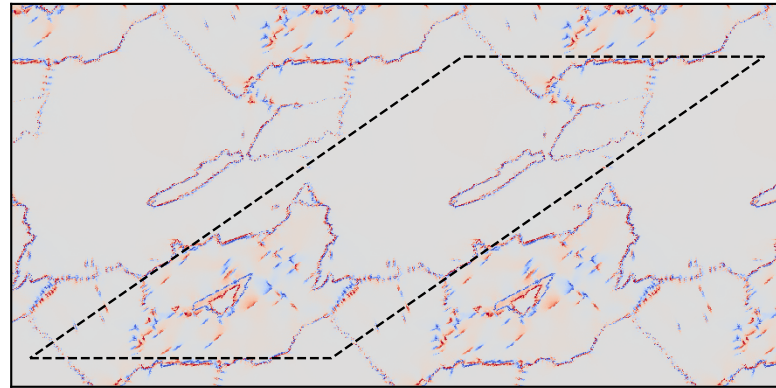
(b) E^{(0)} - E^{(2)}
