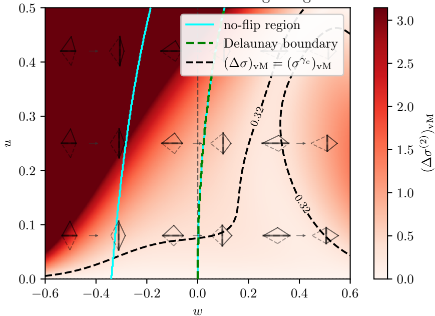
Element 2 von Mises stress-change magnitude
