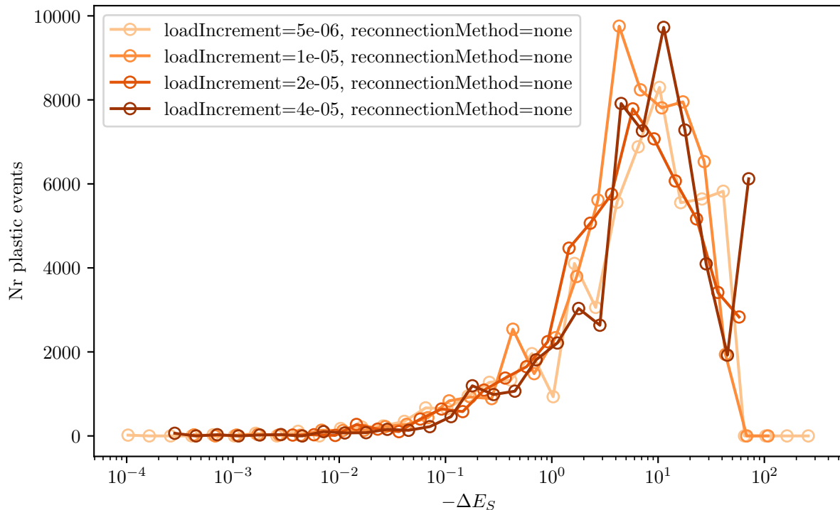
L-BFGS 150x150 1 sample \gamma : 0.15 - 0.14
