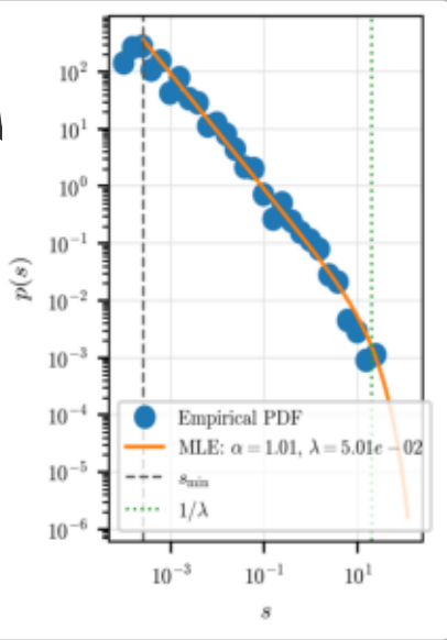
5 MLE \rightarrow \alpha
