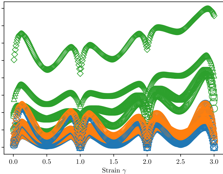
True F
