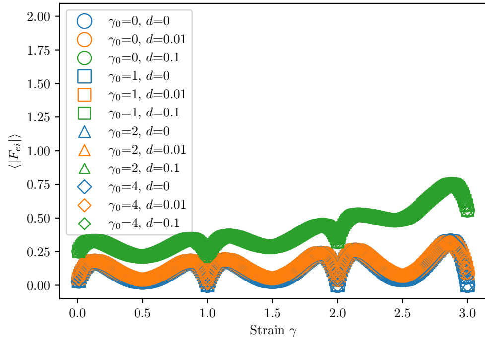
Umut F
