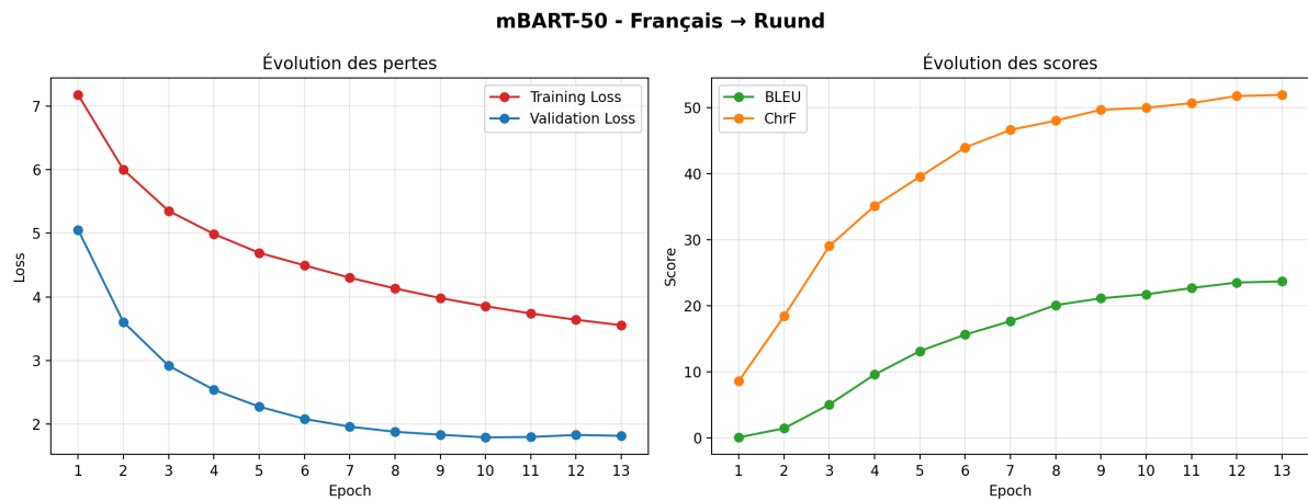
FIGURE 4.4 – Courbes d'entraînement mBART-50 - Français → Ruund
