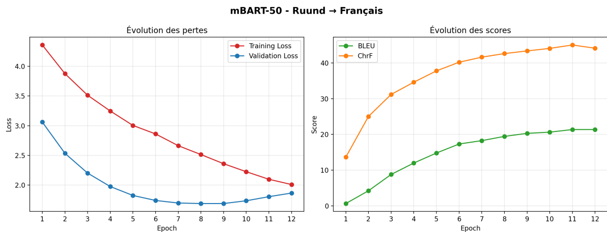
FIGURE 4.5 – Courbes d'entraînement mBART-50 - Ruund → Français
