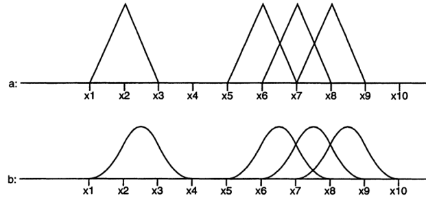
Figure 2: Illustration d'une B-spline isolée et de B-splines chevauchantes, de degré 1 (a) et de degré 2 (b) ( eilers1996 )
