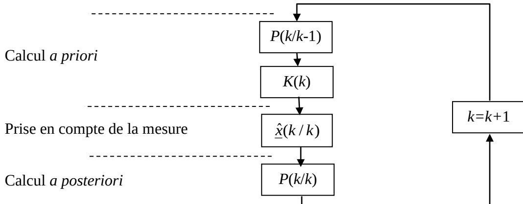
Figure 1.3 : organigramme du filtre de Kalman
