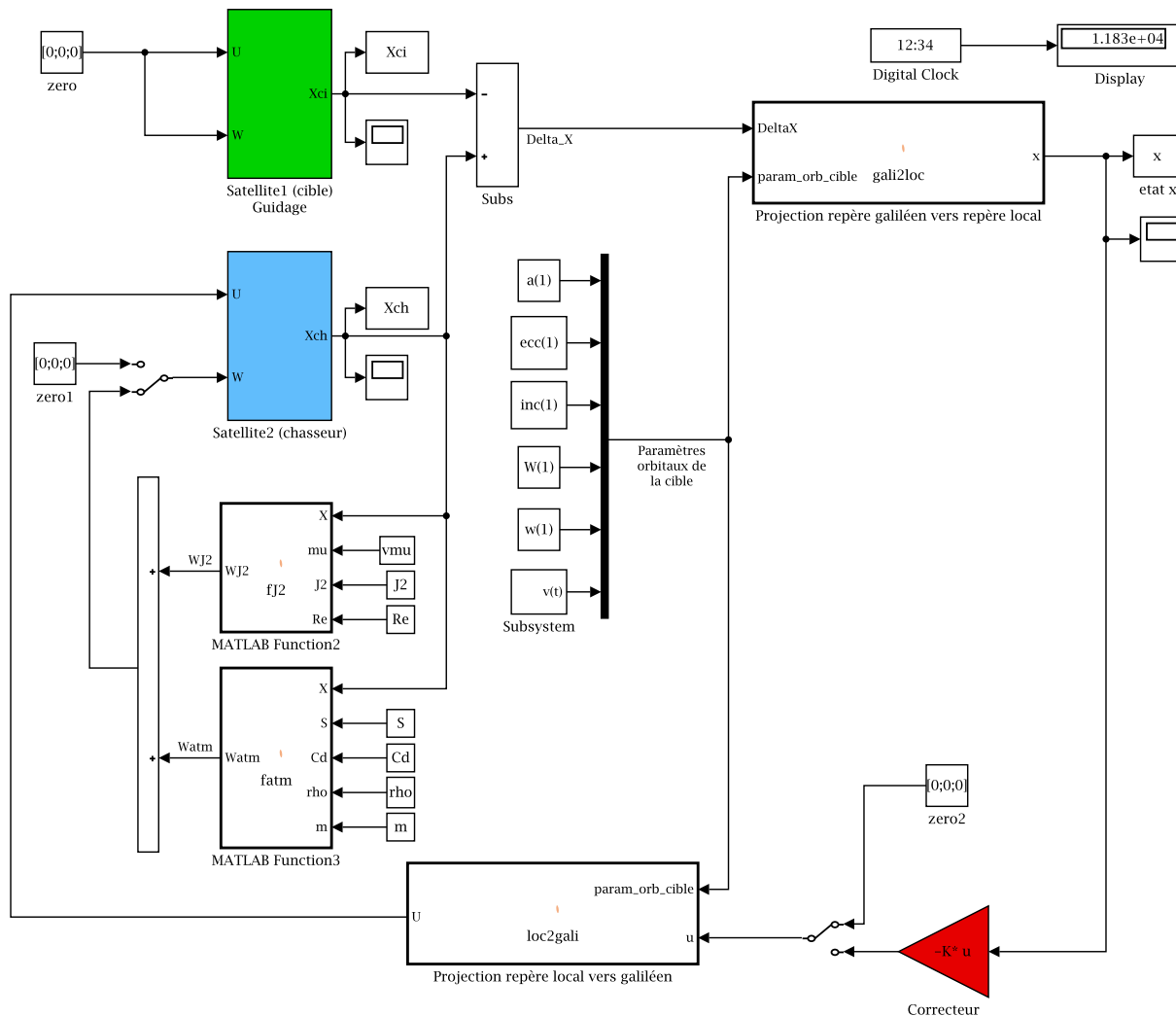
FIGURE 2.3 – Modèle simulink de validation
