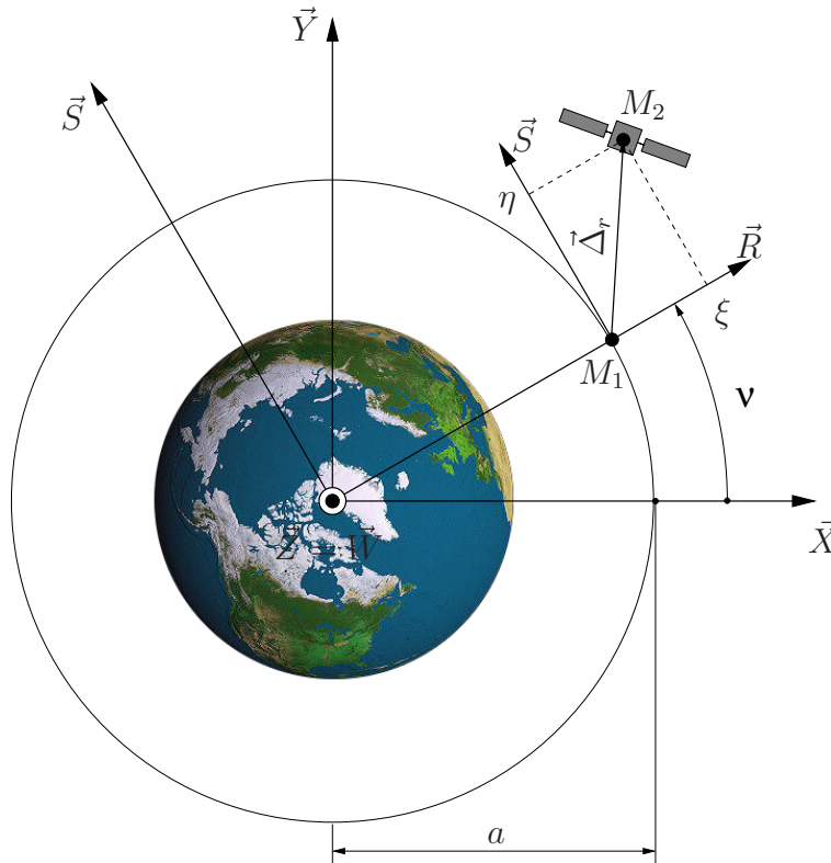
FIGURE 2.2 – Mouvement d'un satellite au voisinage d'une orbite de référence
