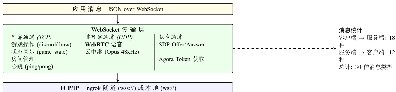
图 4: 通信协议栈
