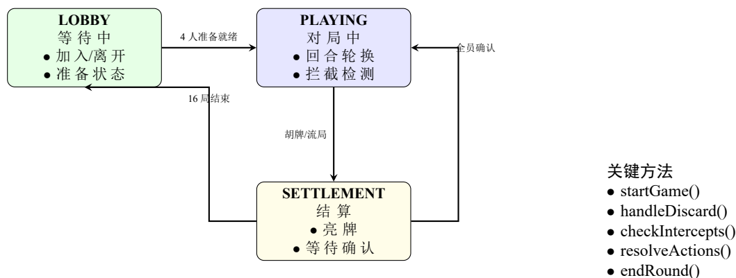
图 7: GameRoom 状态机
