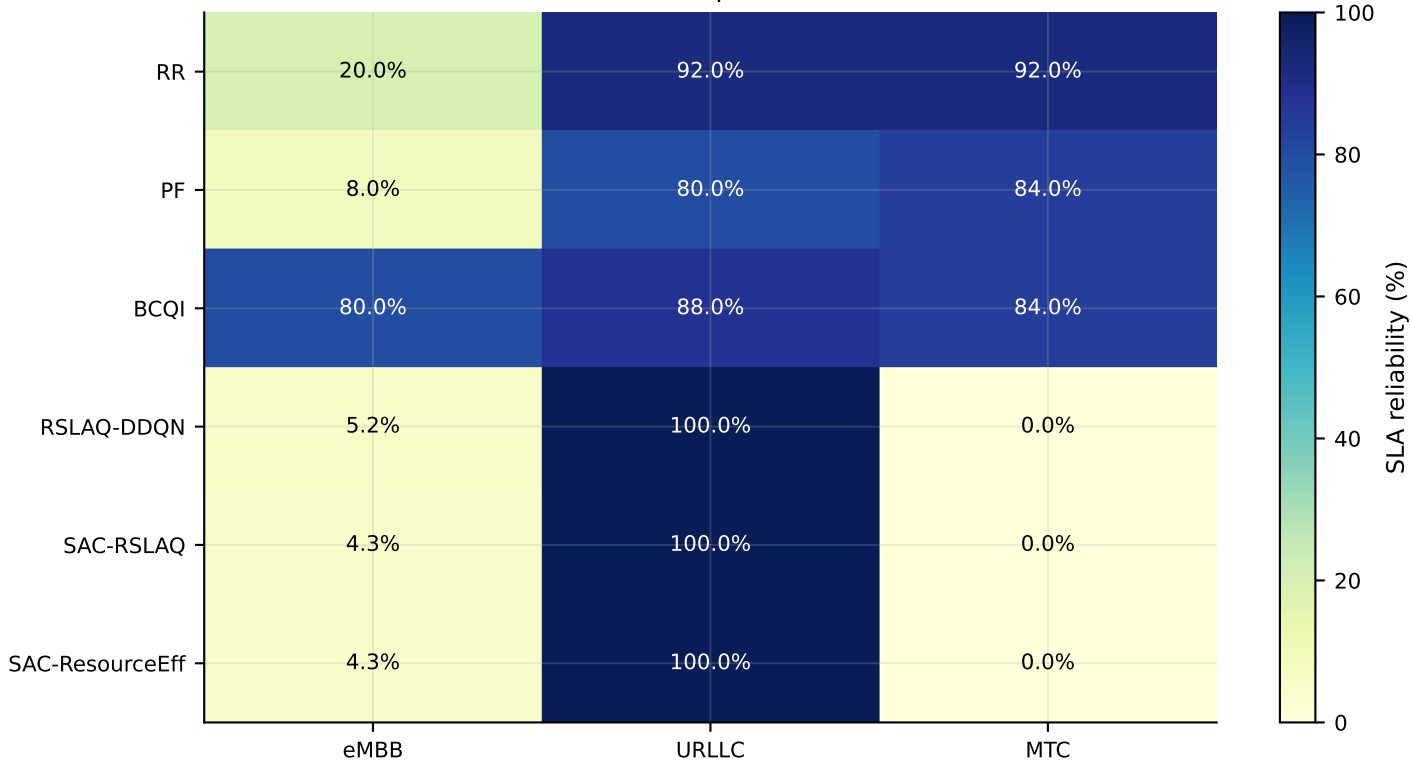
Confiabilidade SLA por metodo e slice
