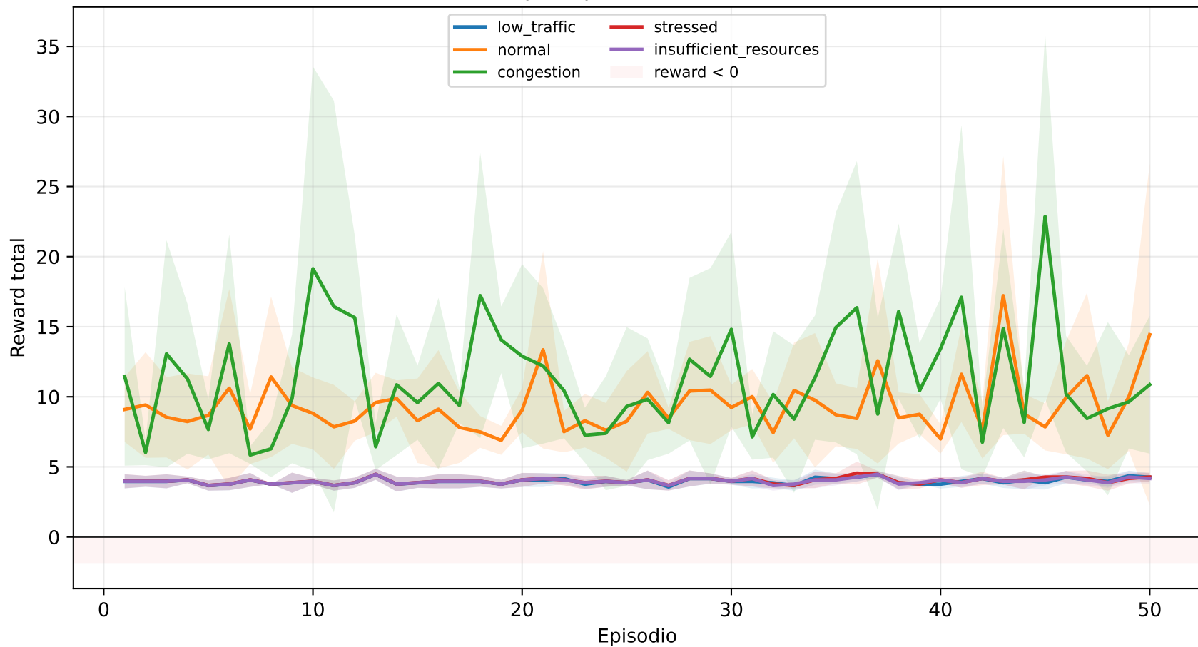
Reward por episodio - RSLAQ/DDQN
