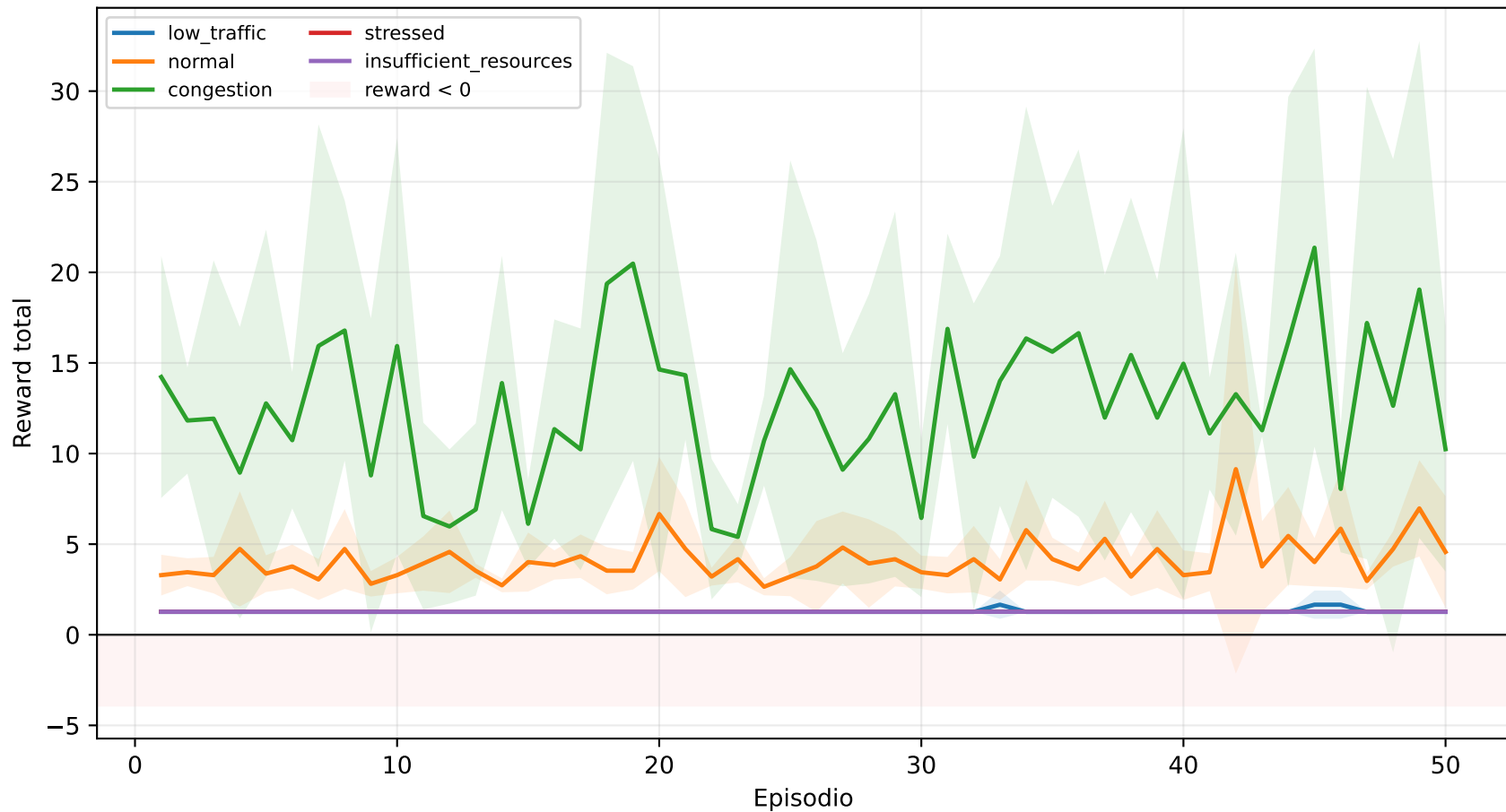
Reward por episodio - SAC
