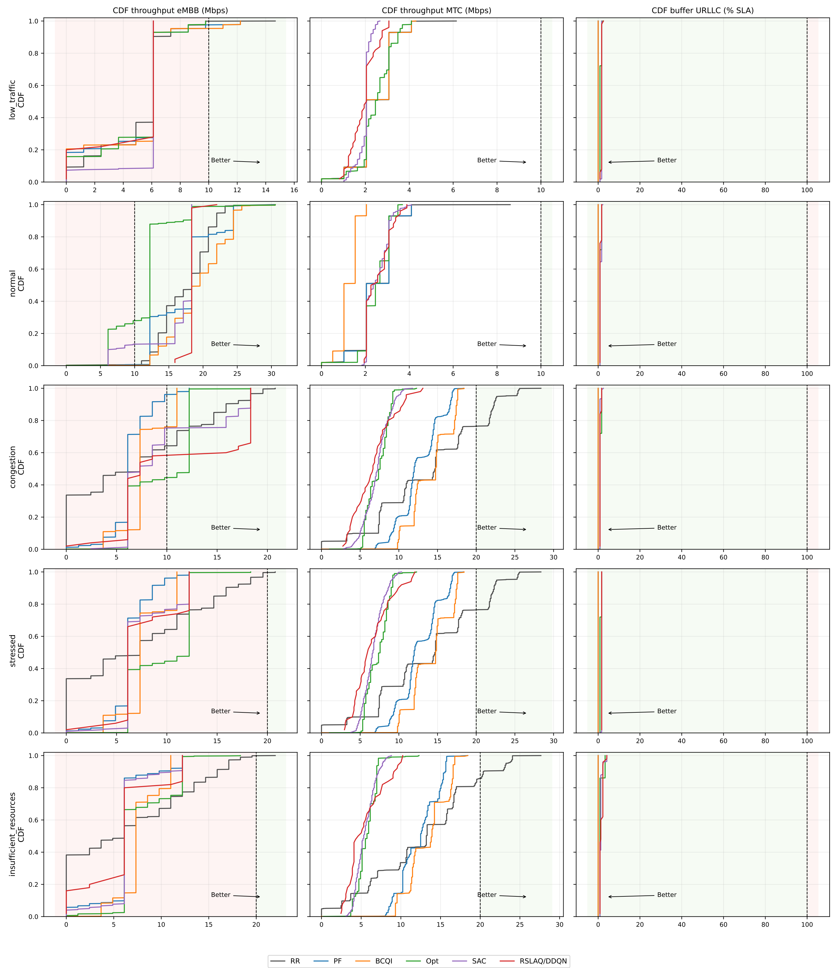
Fig. 6 style - CDFs de KPIs RSLAQ (dados disponíveis)
