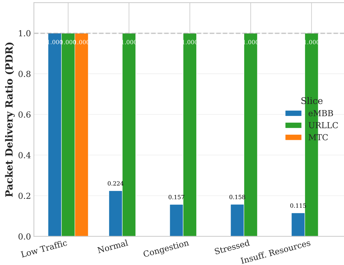
(b) PDR per Slice
