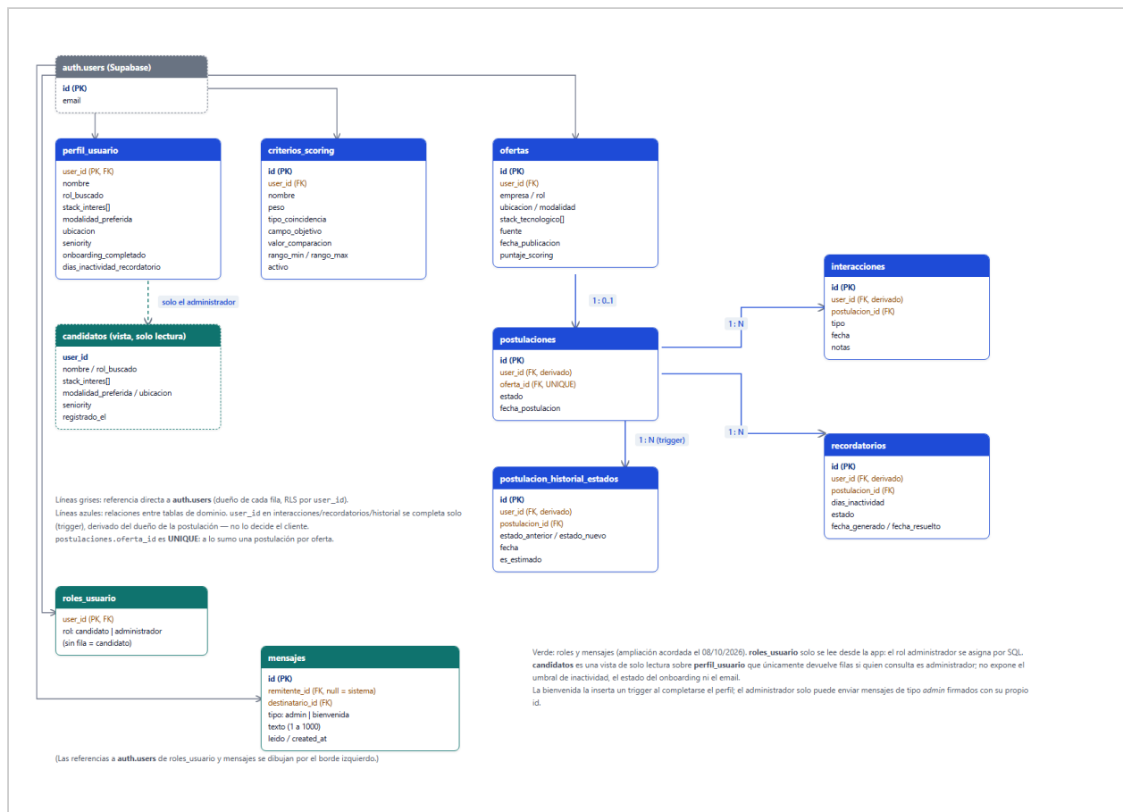
Diagrama entidad-relación del esquema real de Supabase.
