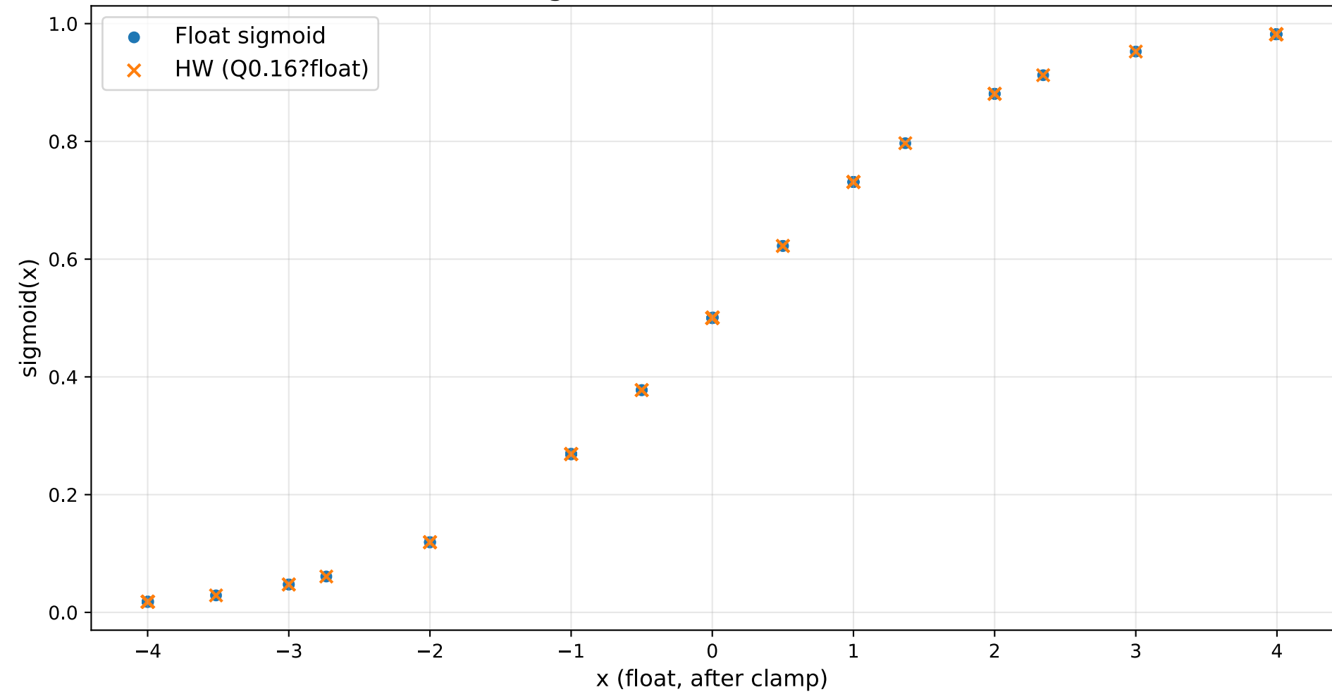
Sigmoid: Float vs HW LUT
