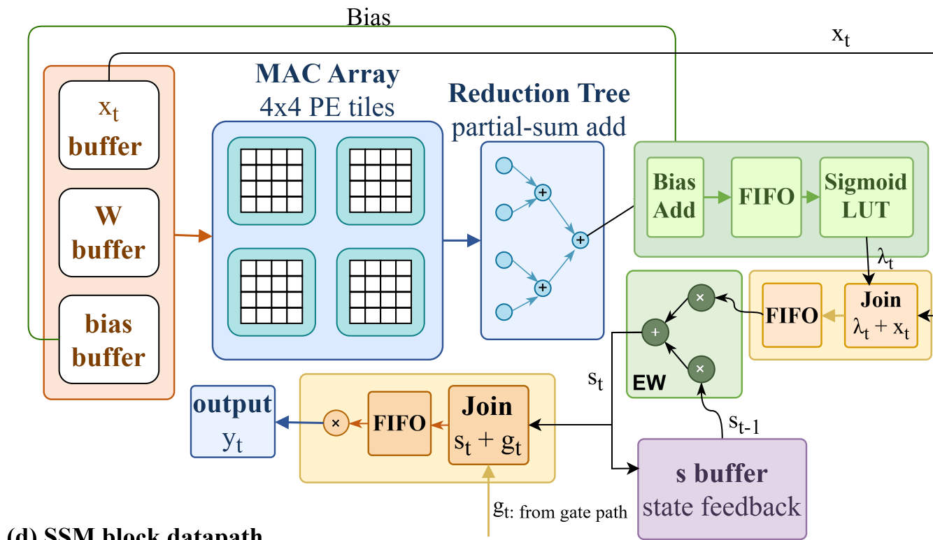
(d) SSM block datapath
