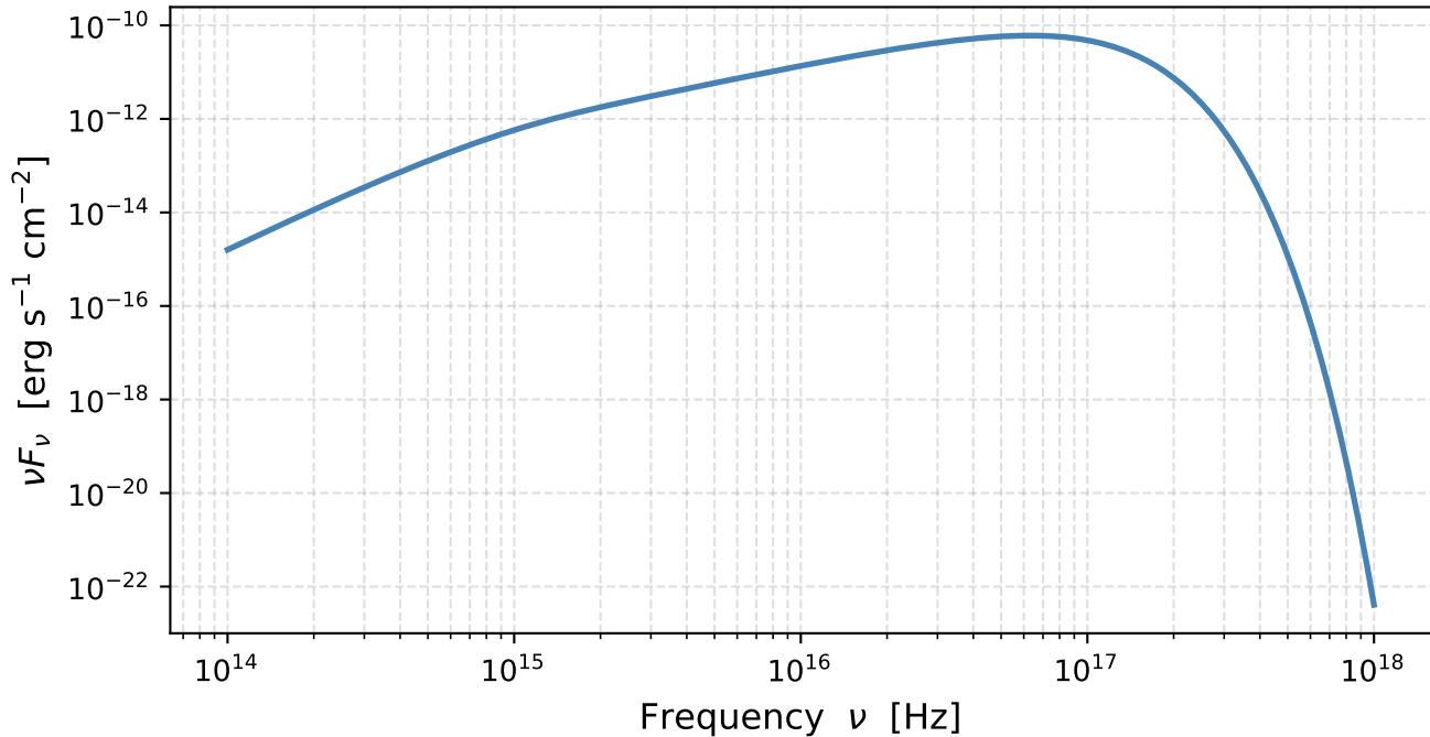
Multi-colour blackbody SED — 10 M_{\odot} BH, \dot{M} = 10^{16} \text{ g s}^{-1} , D_L = 10 \text{ kpc}
