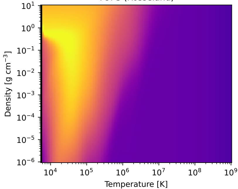
TOPS (Rosseland)
