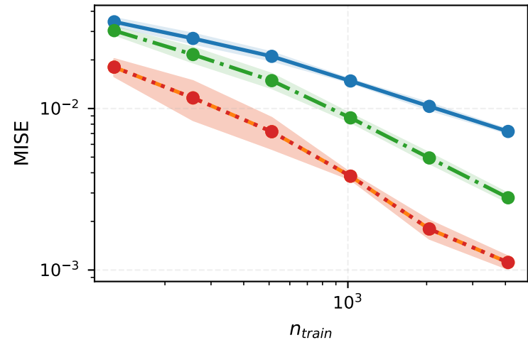
MISE
