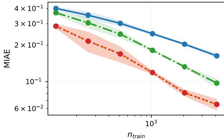
MIAE
