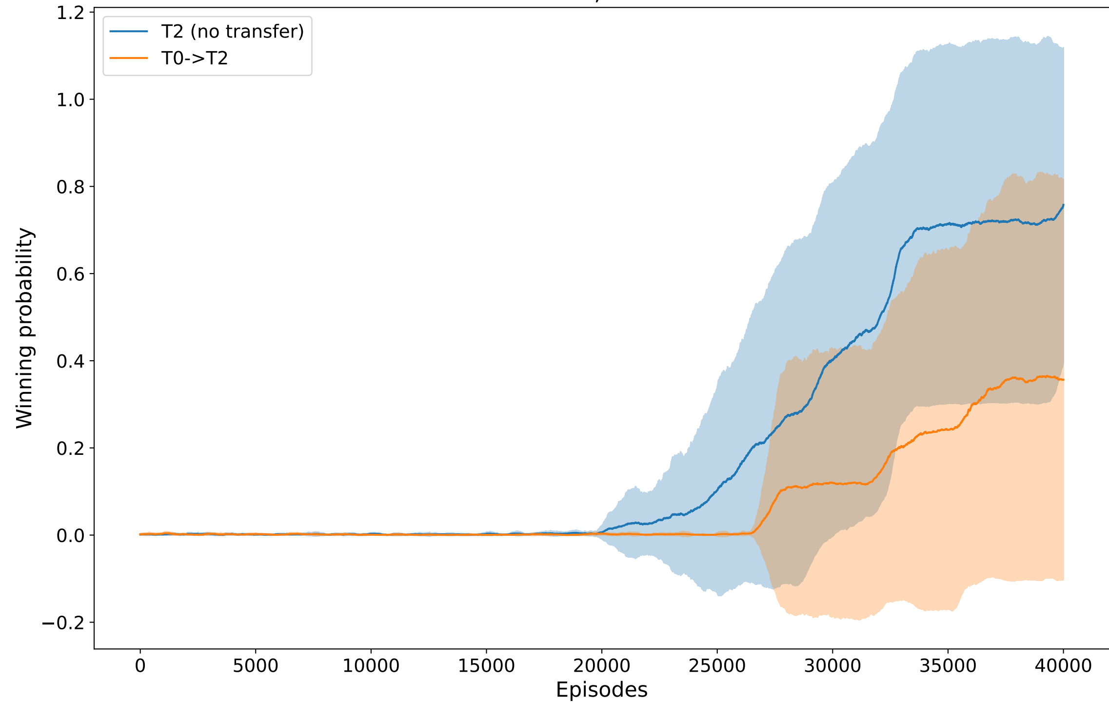
Task 2, Phi V1
