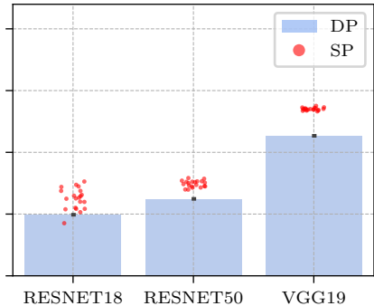
CIFAR100
