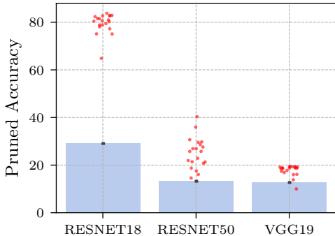
CIFAR10
