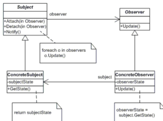
Рис.4 Структура шаблону Observer
