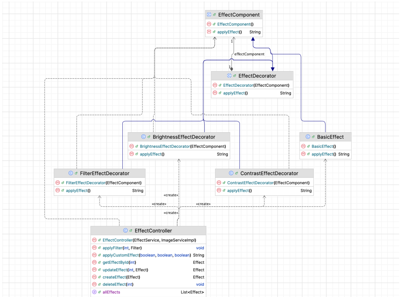
Рис.13 Діаграма класів для патерну Decorator
