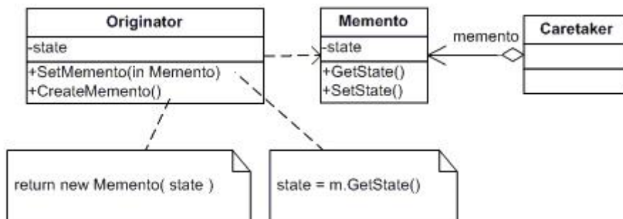
Рис. 3 Структура шаблону Memento
