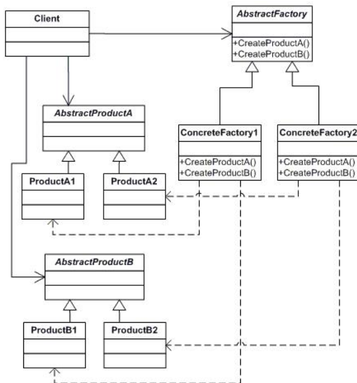
Рис.1 Структура шаблону Abstract Factory
