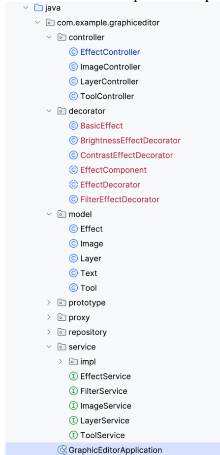
Рис.6 Структура проекту з реалізованими класами
