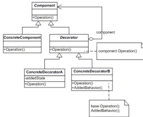
Рис.5 Структура шаблону Decorator
