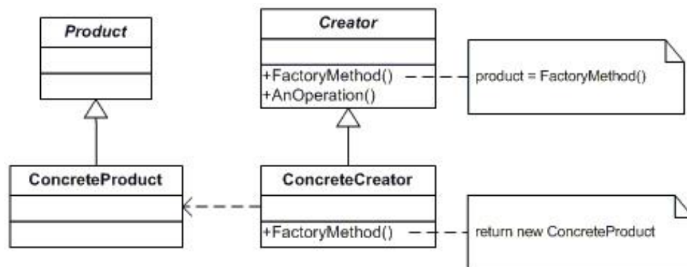
Рис.2 Структура шаблону Factory Method
