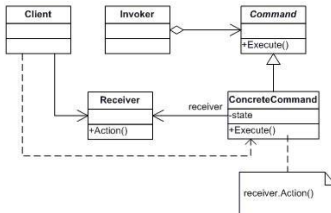
Рис.3 Структура шаблону Command
