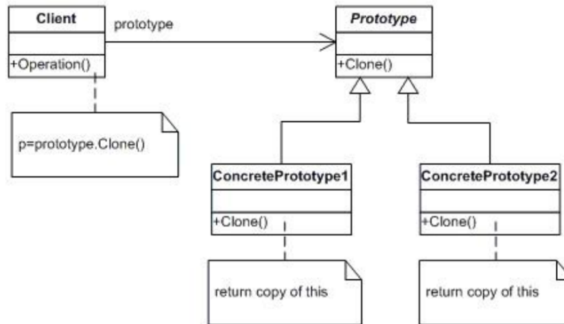
Рис.5 Структура шаблону Prototype
