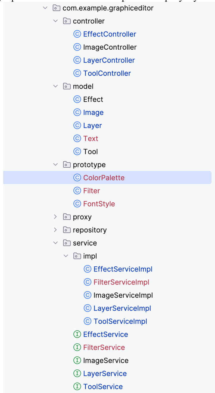
Рис.6 Структура проекту з реалізованими класами
