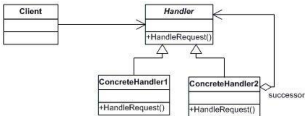
Рис.4 Структура шаблону Chain of Responsibility
