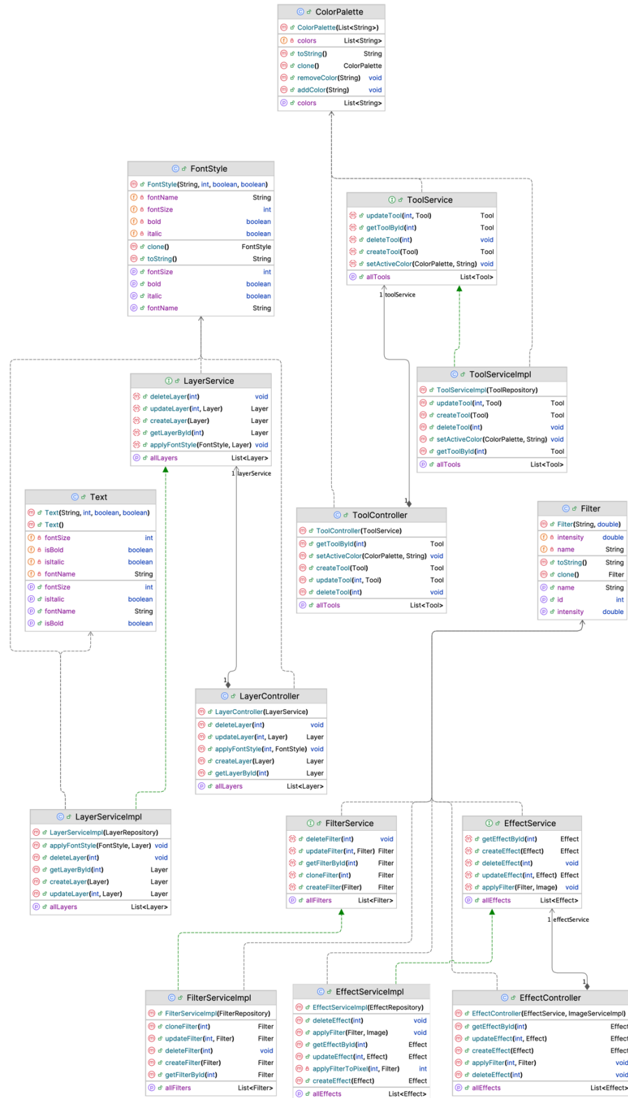
Рис. 10 Діаграма класів для патерну Prototype
