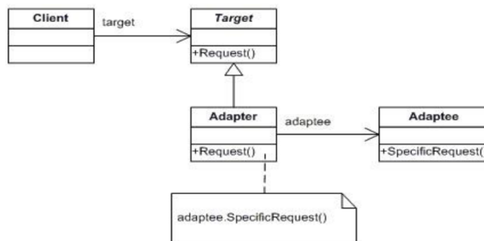
Рис.1 Структура шаблону Adapter
