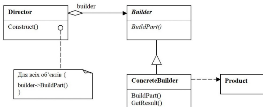
Рис.2 Структура шаблону Builder
