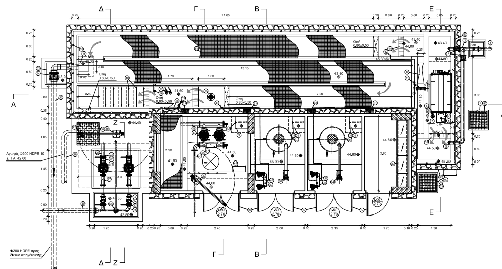
ΚΑΤΟΨΗ Κ/Α 1/50
