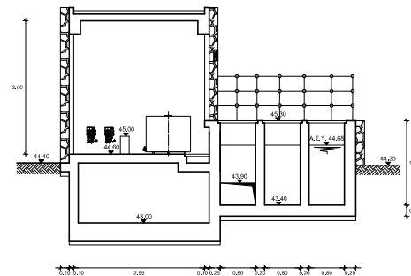
ΤΟΜΗ Β-Β Κ/Α 1/50
