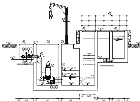
ΤΟΜΗ Δ-Δ Κ/Α 1/50
