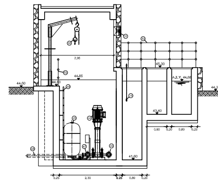
ΤΟΜΗ Γ-Γ Κ/Α 1/50
