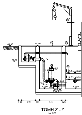
ΤΟΜΗ Ζ-Ζ Κ/Α 1/50
