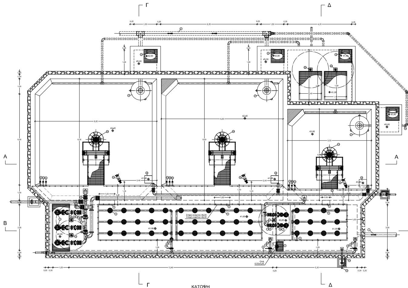
ΚΑΤΟΨΗ ΚΑ. 150
