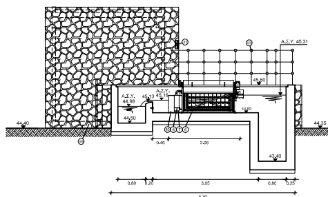
ΤΟΜΗ Ε-Ε Κ/Α 1/50
