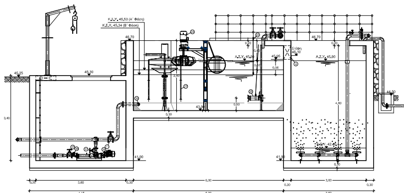
ΤΟΜΗ Δ - Δ ΚΑ. 1/50
