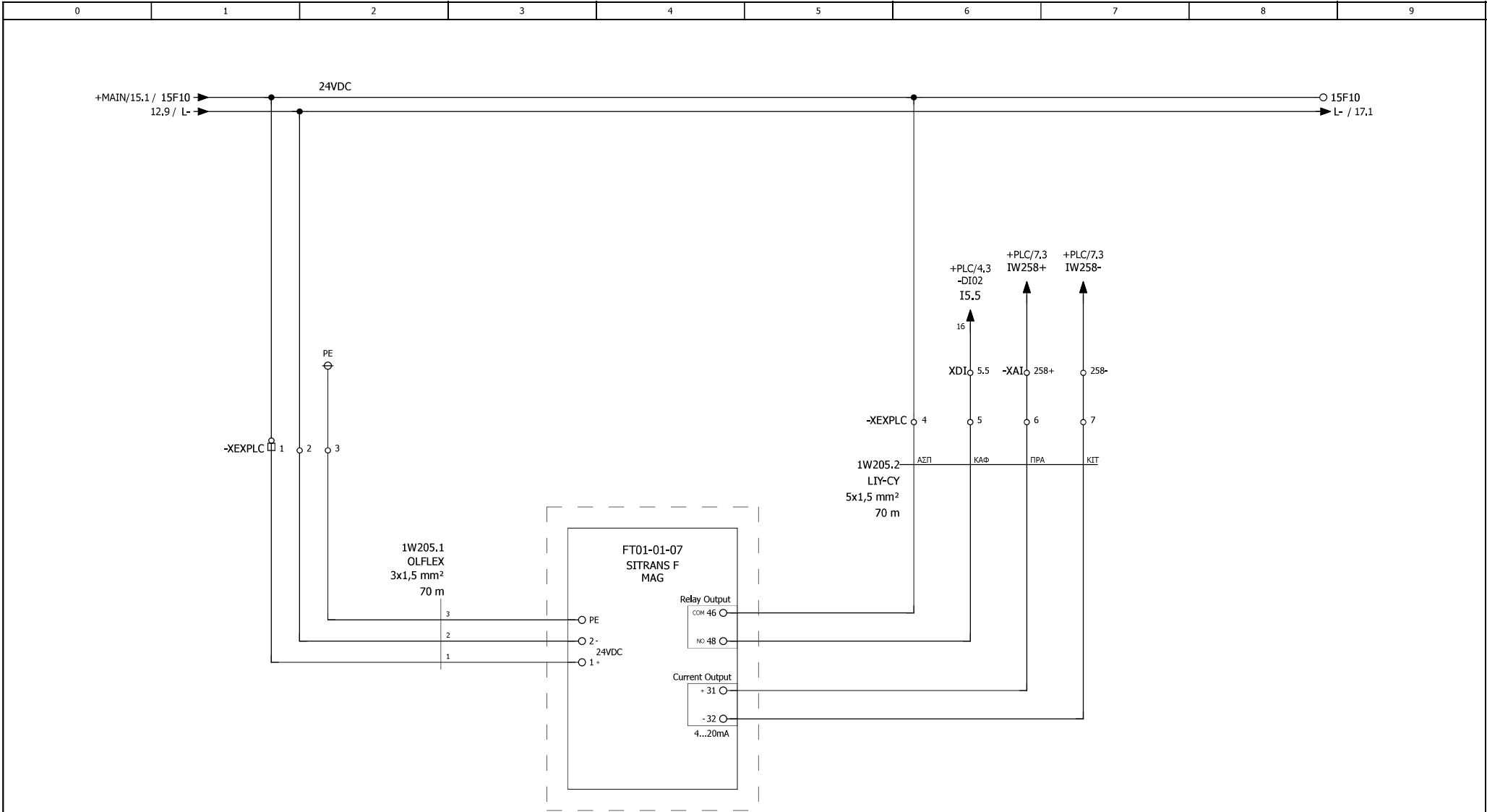
ΗΛΕΚΤΡΟΜΑΓΝΗΤΙΚΟΣ ΜΕΤΡΗΤΗΣ ΠΑΡΟΧΗΣ ΕΙΣΟΔΟΥ
