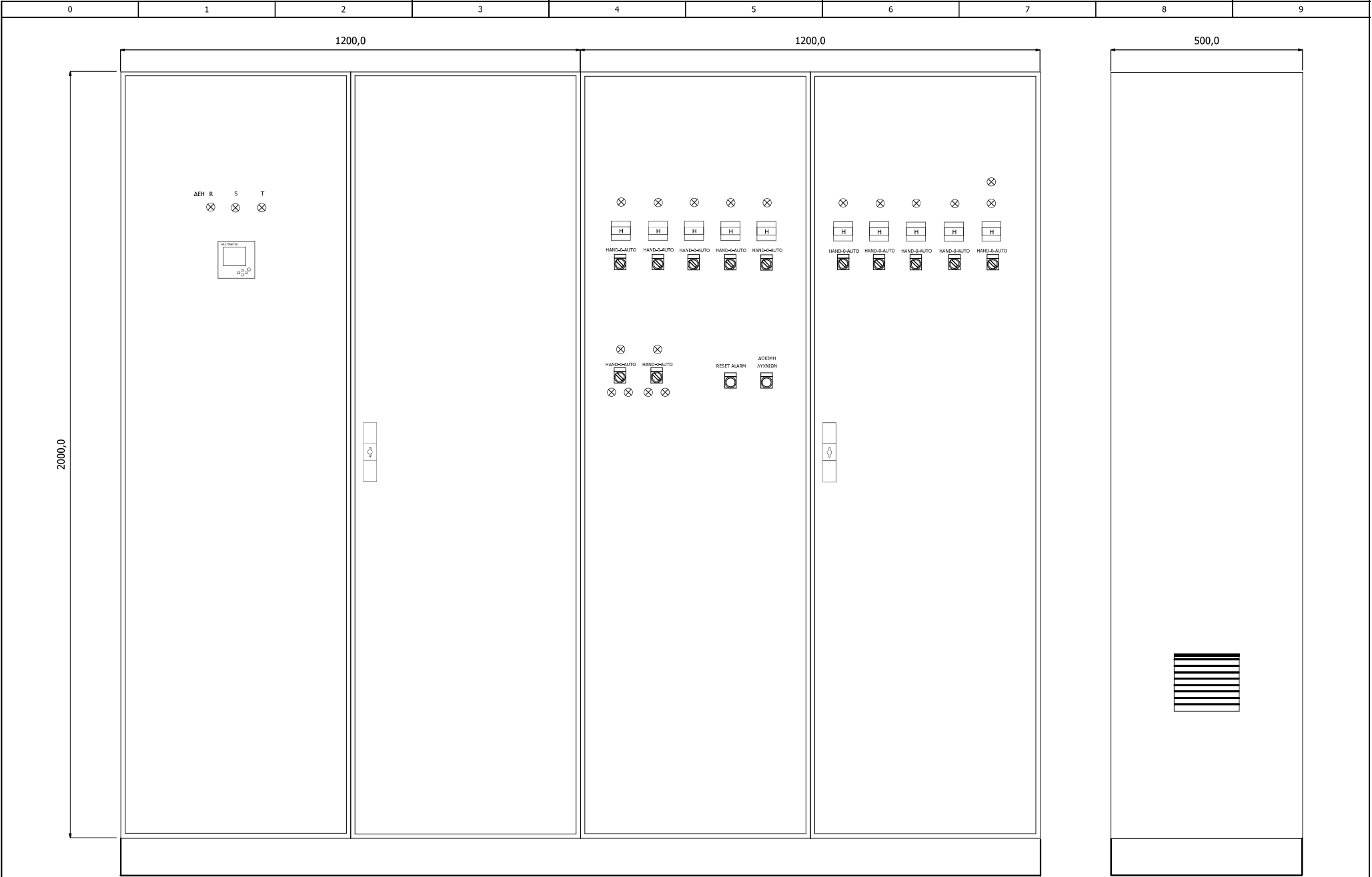
ΠΡΟΣΟΨΗ & ΠΛΑΪΝΗ ΟΨΗ ΗΛΕΚΤΡΙΚΟΥ ΠΙΝΑΚΑ MCC1 (HxWxD) (2000mm x 2400mm x 500mm)
