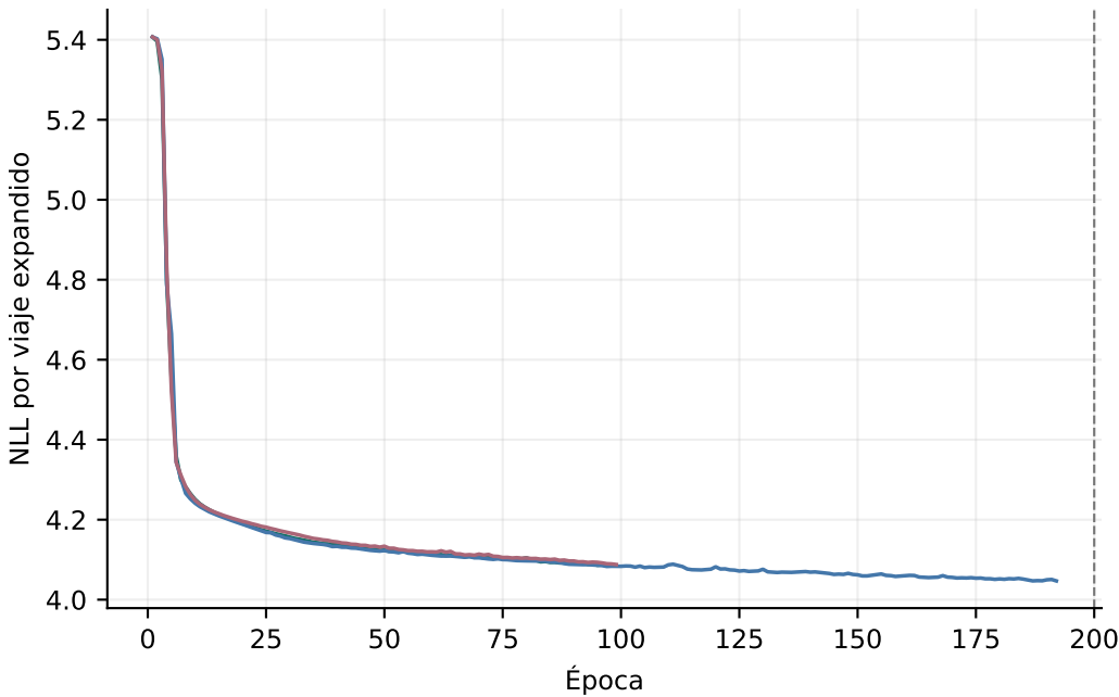
H3-r8 · pérdida de entrenamiento
