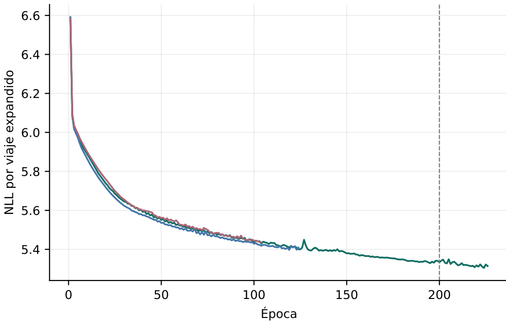
H3-r7 · pérdida de entrenamiento
