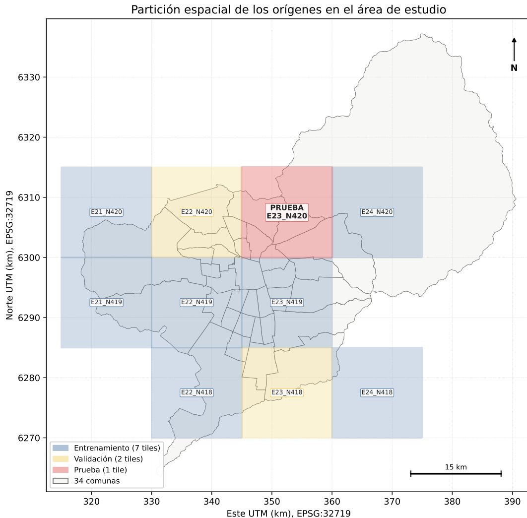
Figura 7: Ubicación de los diez tiles de 15 km sobre el área de estudio y rol de cada bloque en la partición de orígenes. Las etiquetas E{e}_N{n} codifican los índices Este y Norte de cada bloque en la cuadrícula UTM. El bloque de prueba E23_N420 se destaca en rojo; los destinos de todo el dominio permanecen disponibles en las tres particiones. Fuente: elaboración propia a partir del dominio territorial aprobado y la agenda congelada de particiones.
