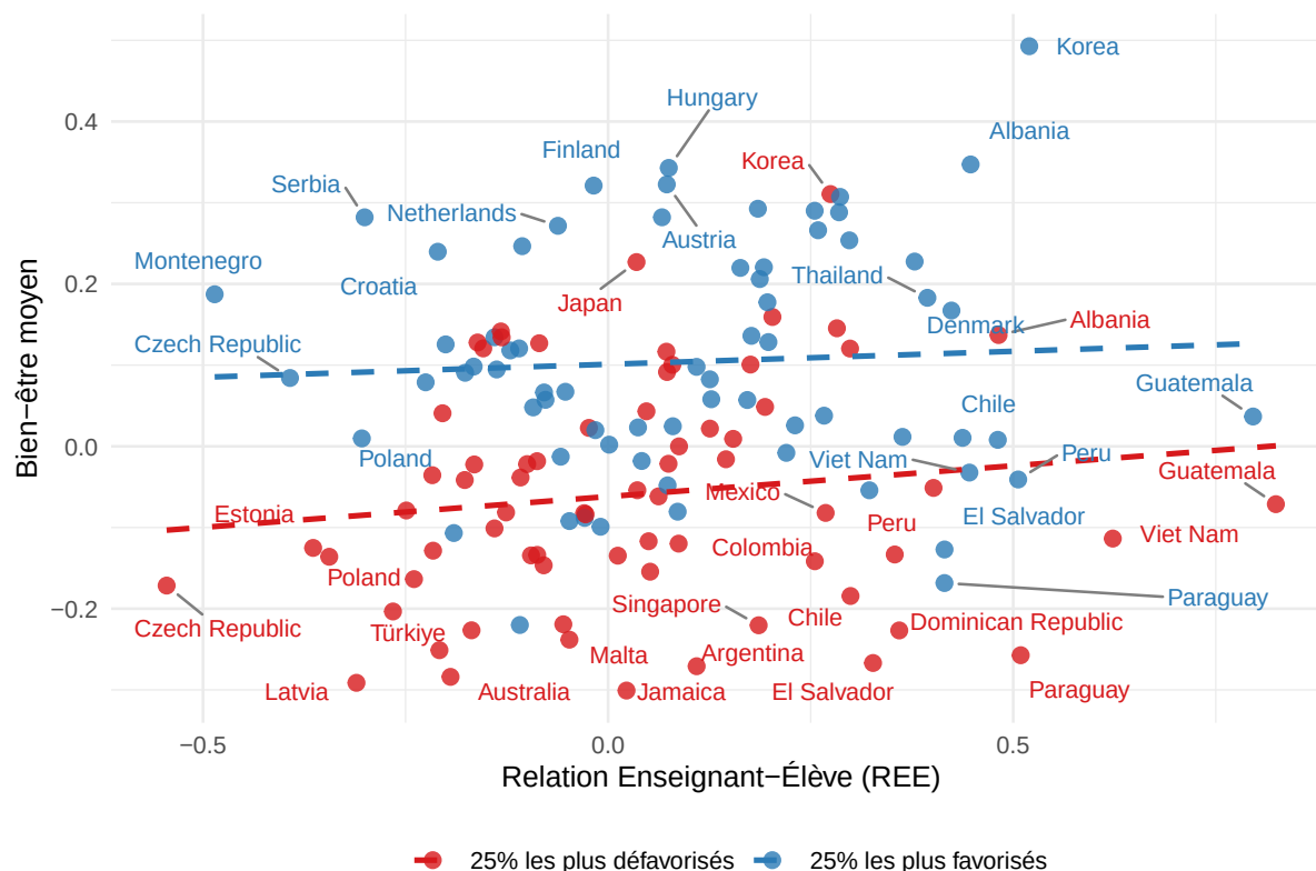
FIGURE 18 – Nuage de points représentant la REE et bien-être par pays selon la catégorie ESCS
