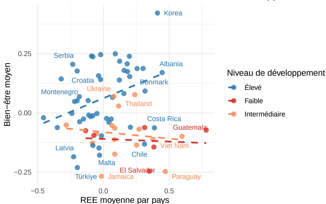
FIGURE 16 – Nuage de points représentant la REE des élèves en fonction de leur bien-être regroupés par pays et différenciés selon leur niveau de développement
