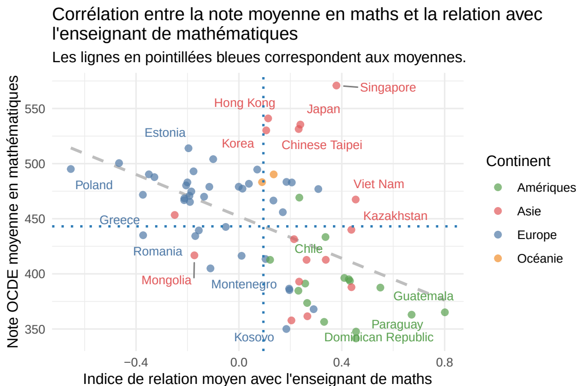
FIGURE 6 – Nuage de points représentant la corrélation entre la note moyenne en mathématiques et la relation avec le professeur de cette matière par pays
