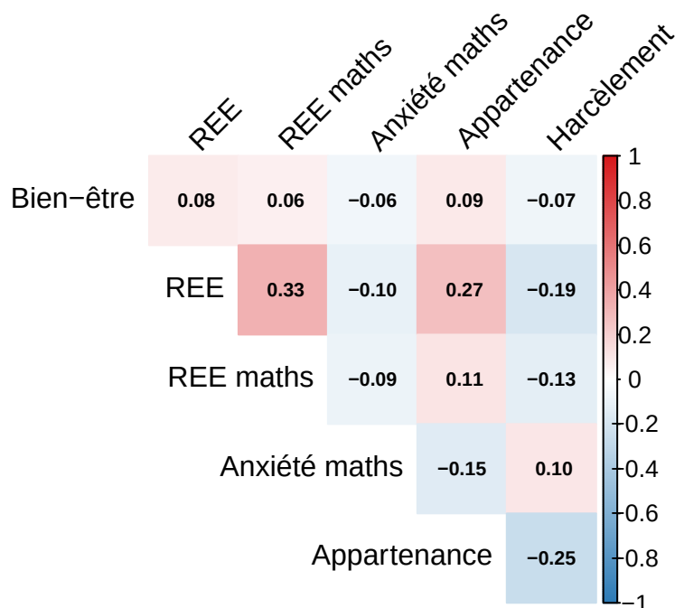
FIGURE 14 – Matrice de corrélation entre la variable REE et les variables de bien-être
