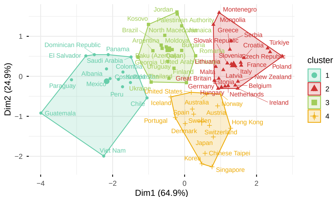
FIGURE 12 – Regroupement des pays selon la méthode du k-means
