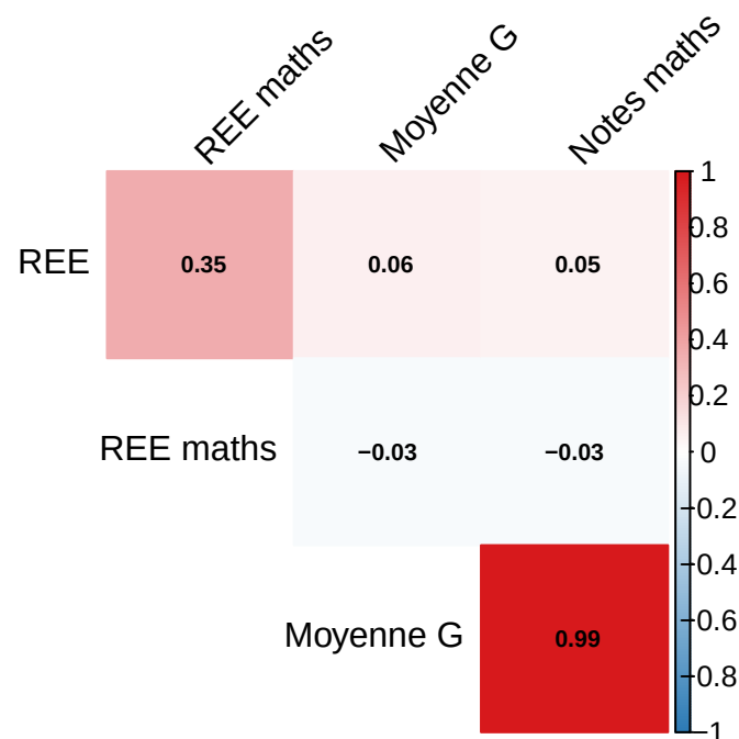
FIGURE 5 – Matrice de corrélation entre les variables
