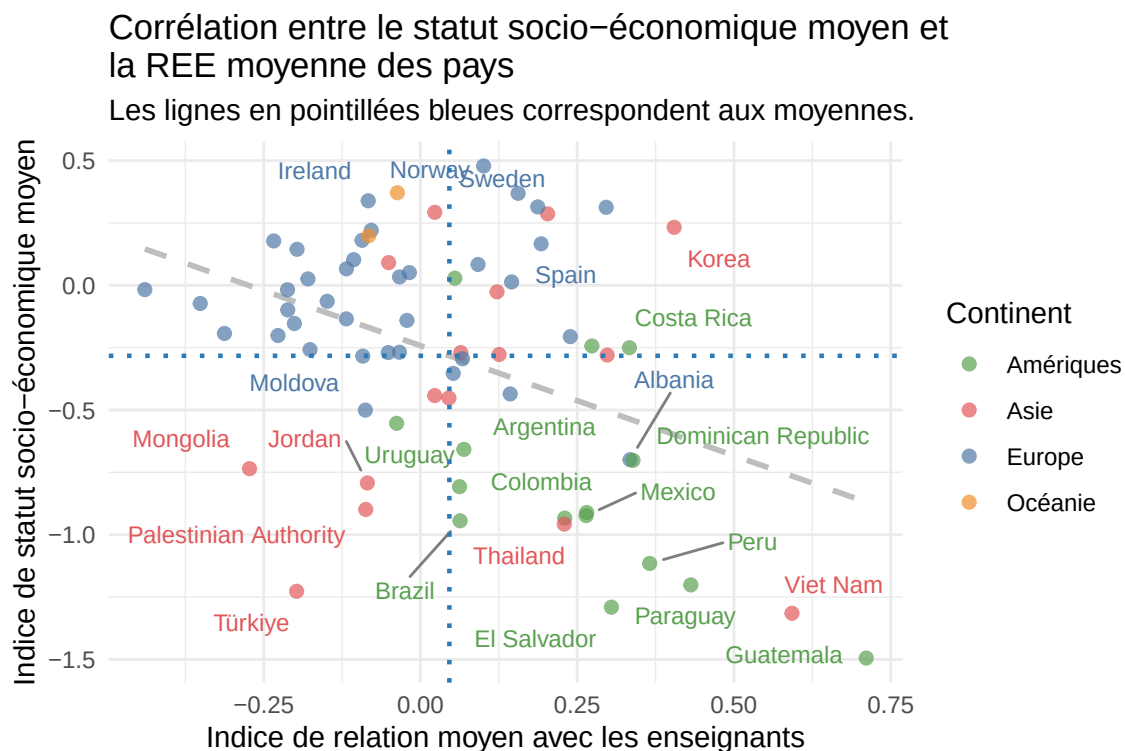
FIGURE 9 – Nuage de points représentant les pays en fonction de leur REE moyen et de leur statut socio-économique
