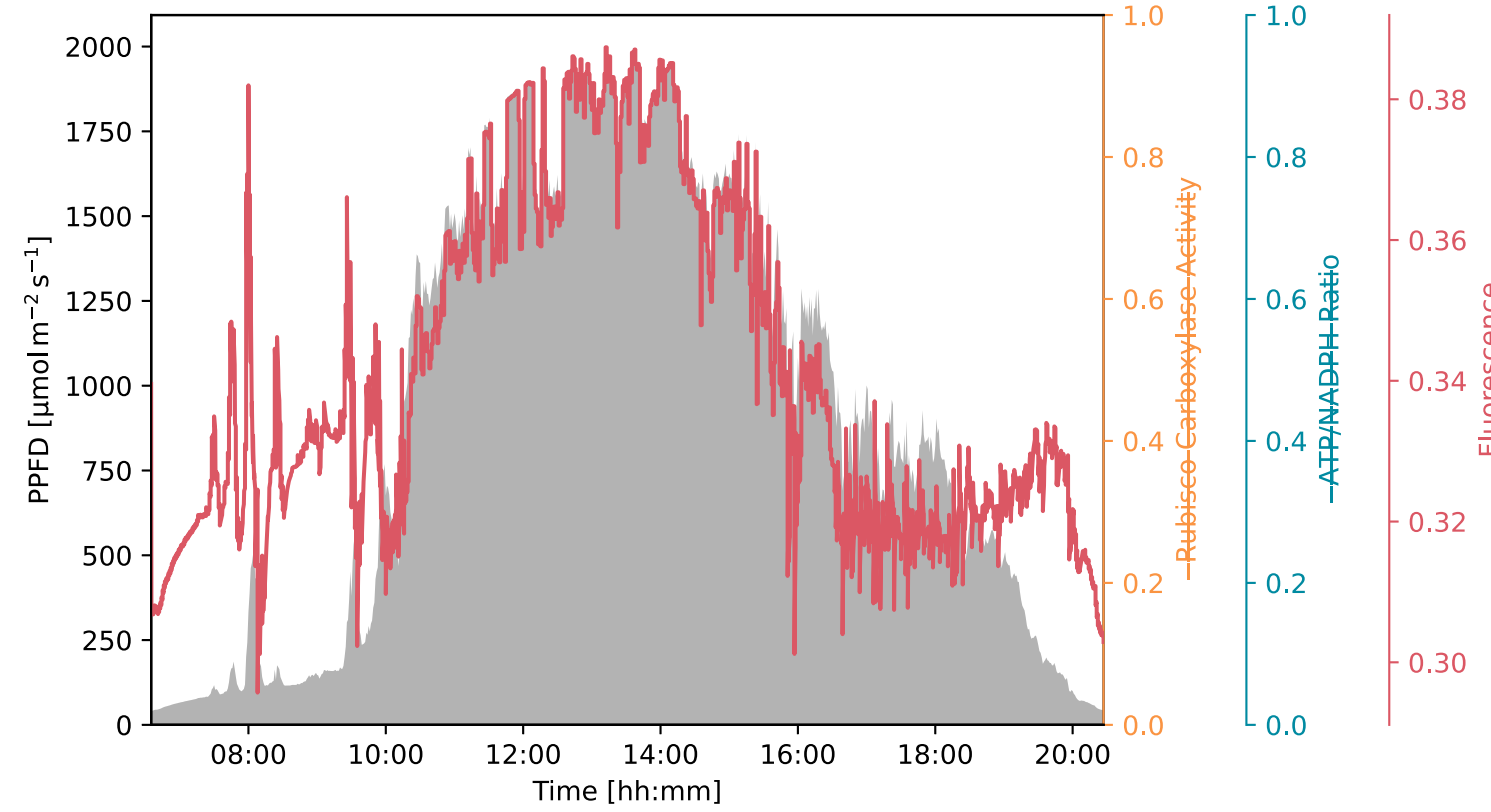
Fuente2024
