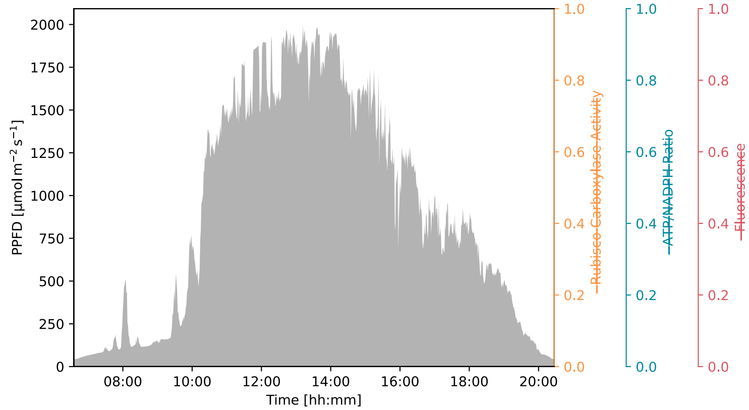
Saadat2021
