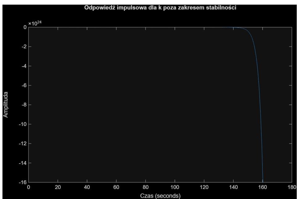
Rysunek 8: Charakterystyka impulsowa dla k = -15
