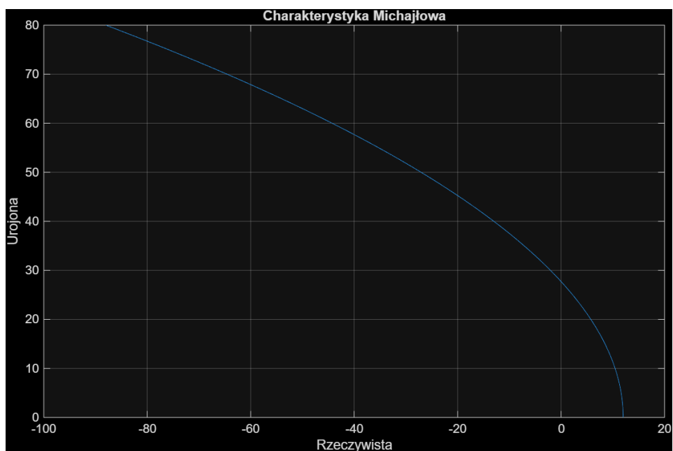
Rysunek 7: Charakterystyka Michajłowa
