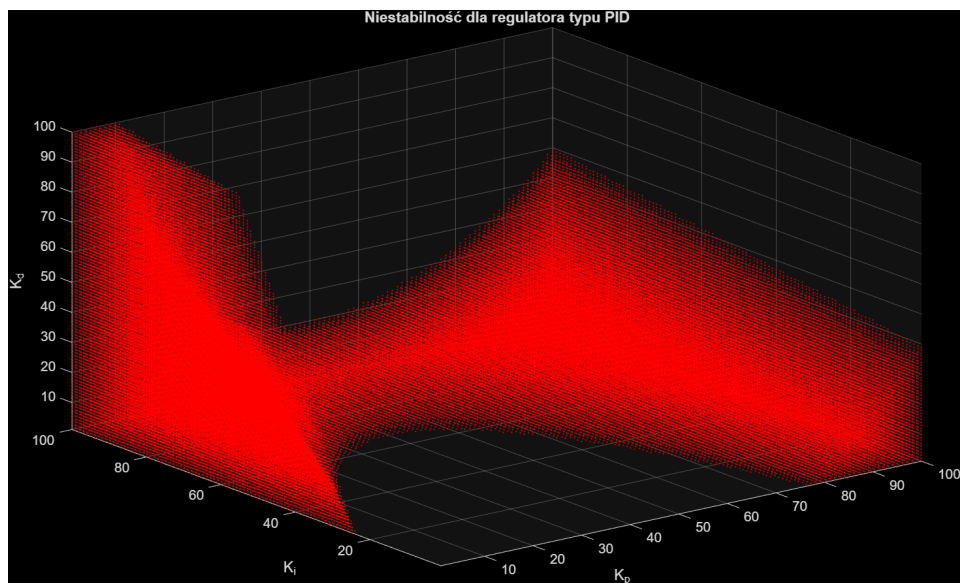
Rysunek 14: Wykres stabilności dla regulatora PID bez punktów oznaczających stabilność
