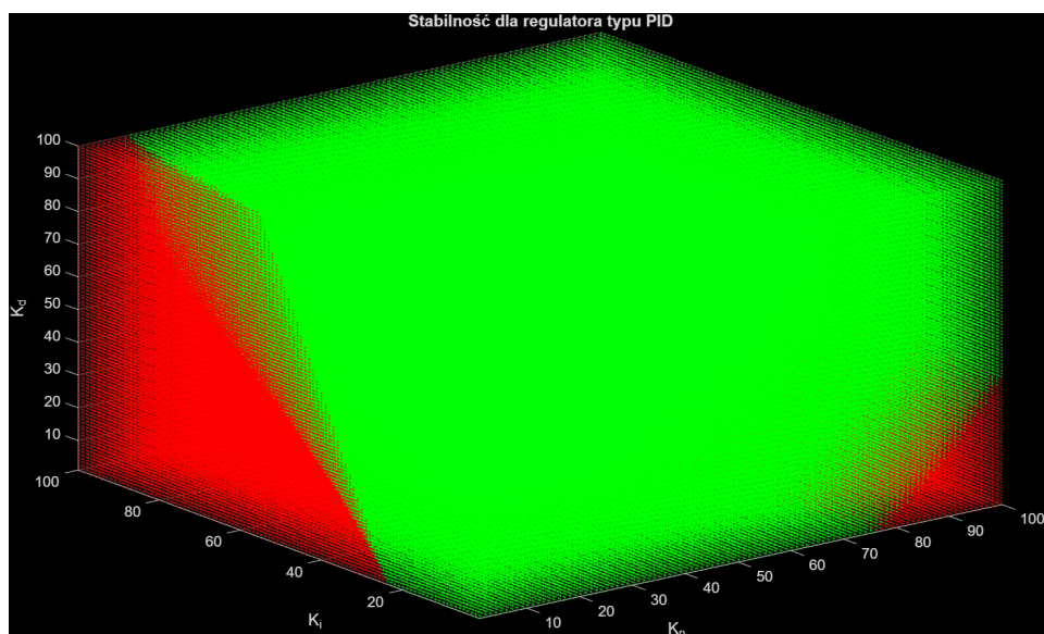
Rysunek 13: Wykres stabilności dla regulatora PID
