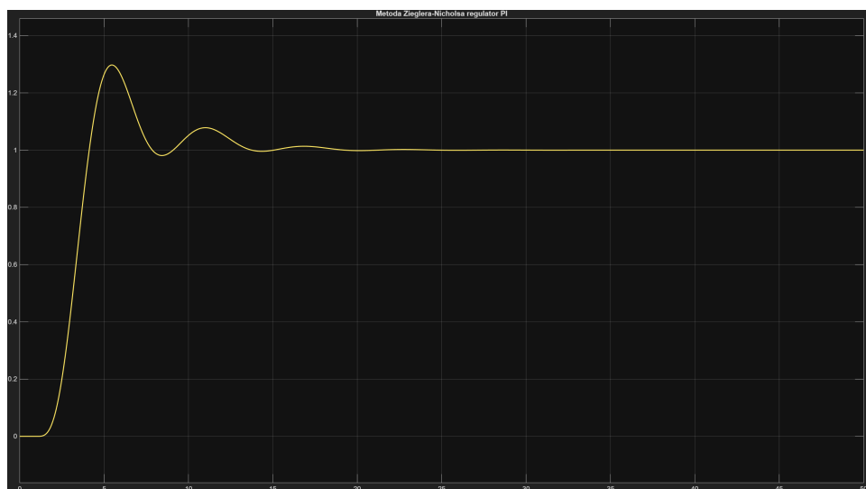
Rysunek 16: Charakterystyka skokowa dla metody Zieglera-Nicholsa dla regulatora typu PI
