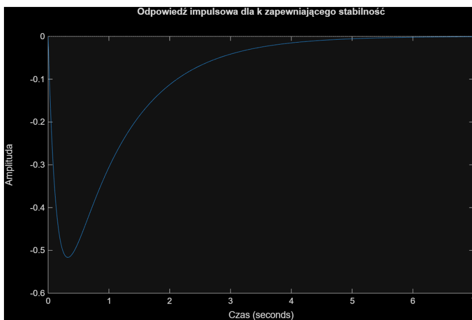
Rysunek 10: Charakterystyka impulsowa dla k = -5
