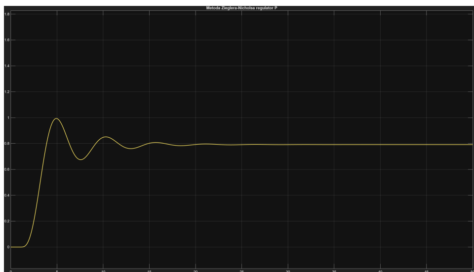
Rysunek 15: Charakterystyka skokowa dla metody Zieglera-Nicholsa dla regulatora typu P
