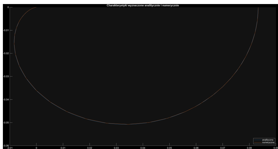
Rysunek 6: Charakterystyki nyquista wyznaczone metodą analityczną i numeryczną
