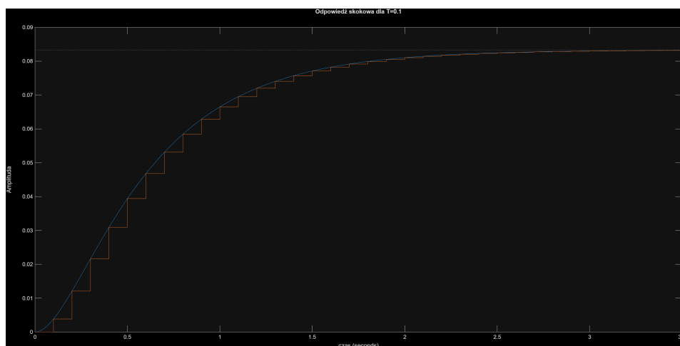
Rysunek 19: Odpowiedź skokowa obiektów dla T=0.1
