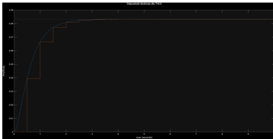
Rysunek 20: Odpowiedź skokowa obiektów dla T=0.5
