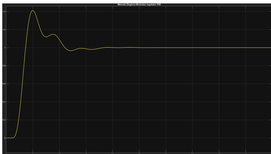
Rysunek 17: Charakterystyka skokowa dla metody Zieglera-Nicholsa dla regulatora typu PID
