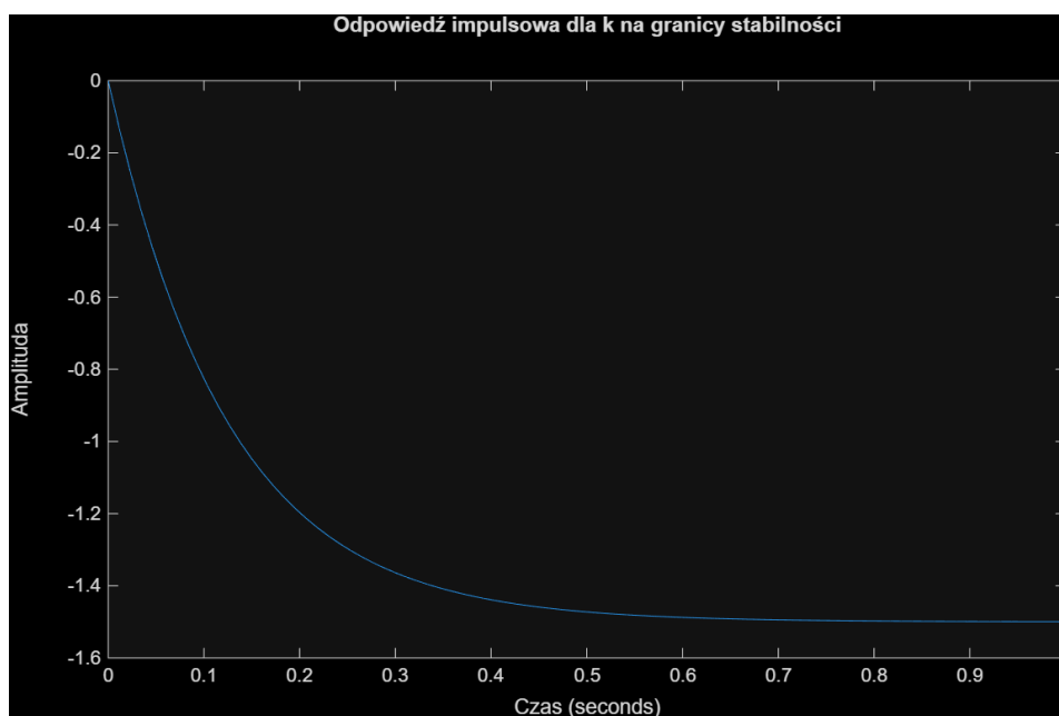
Rysunek 9: Charakterystyka impulsowa dla k = -12
