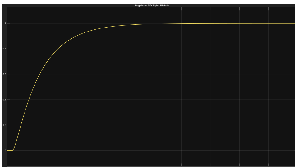
Rysunek 7: Charakterystyka skokowa dla metody Zieglera-Nicholsa dla regulatora typu PID
