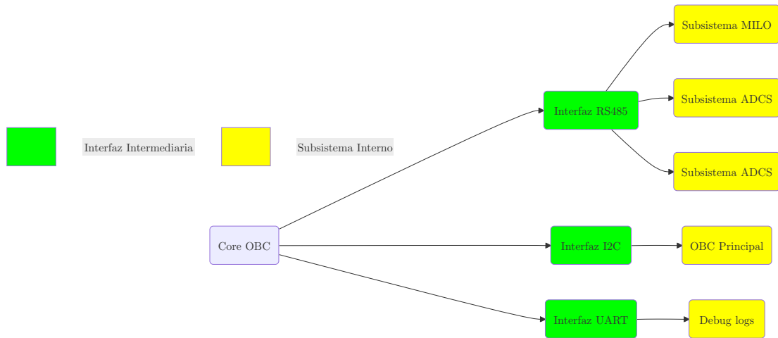
Figura 4: Arquitectura de la OBC secundaria. Elaboración propia.
