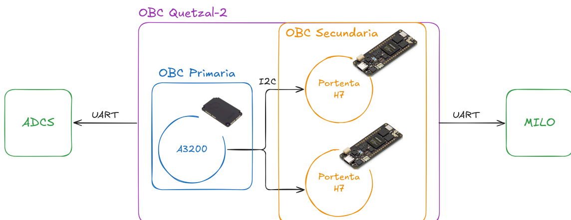
Figura 3: Diagrama de componentes de la OBC y sus protocolos de comunicación.
