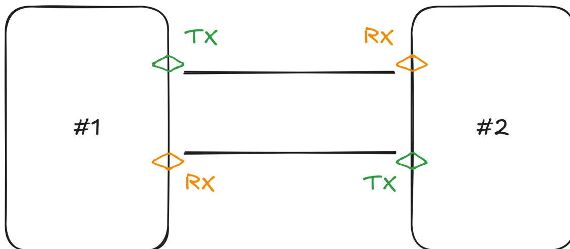
Figura 4: Diagrama de conexión de pines entre dos dispositivos que soportan el protocolo de comunicación UART.
