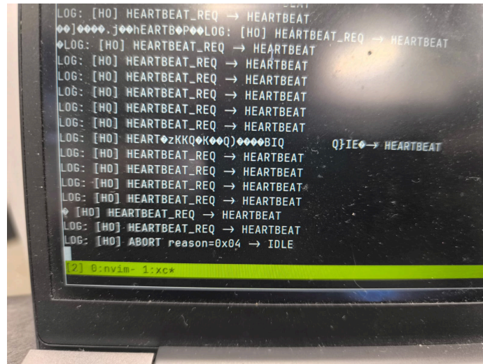
Figura 6: Prueba del protocolo de handover corriendo con hardware real entre la computadora primaria y secundaria. Logs desde la perspectiva de la OBC secundaria.
